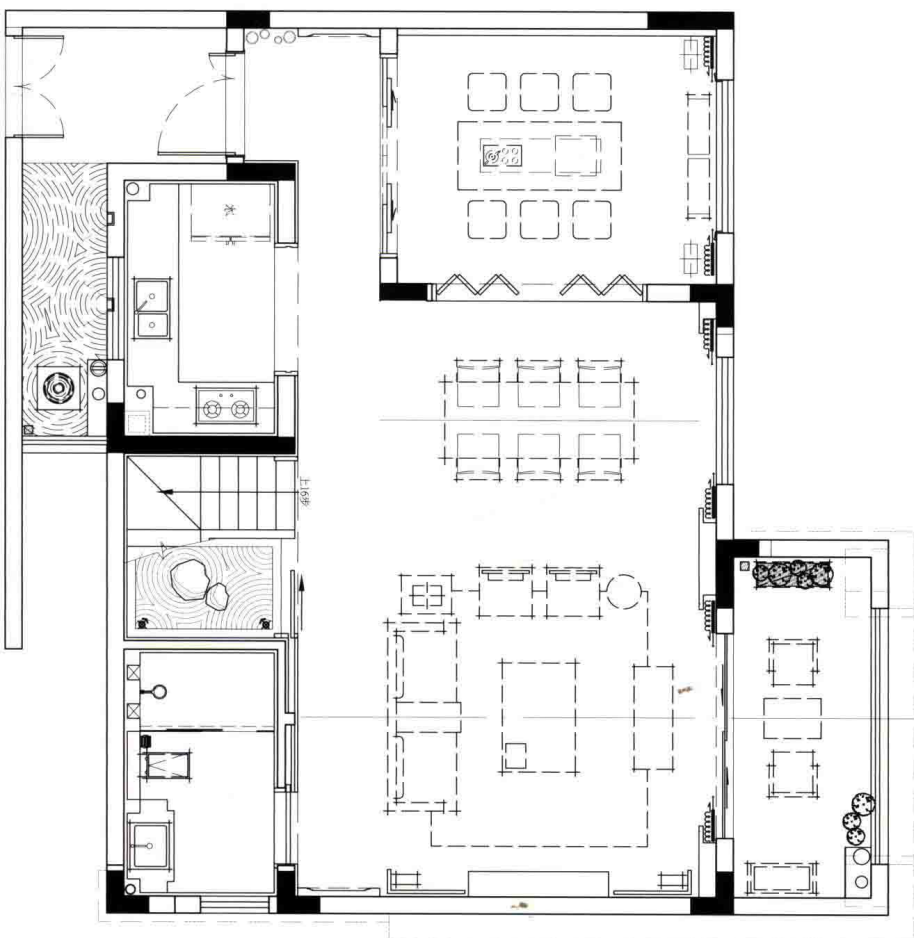
一层平面图
