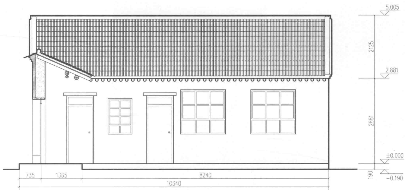
东厦房西立面图
