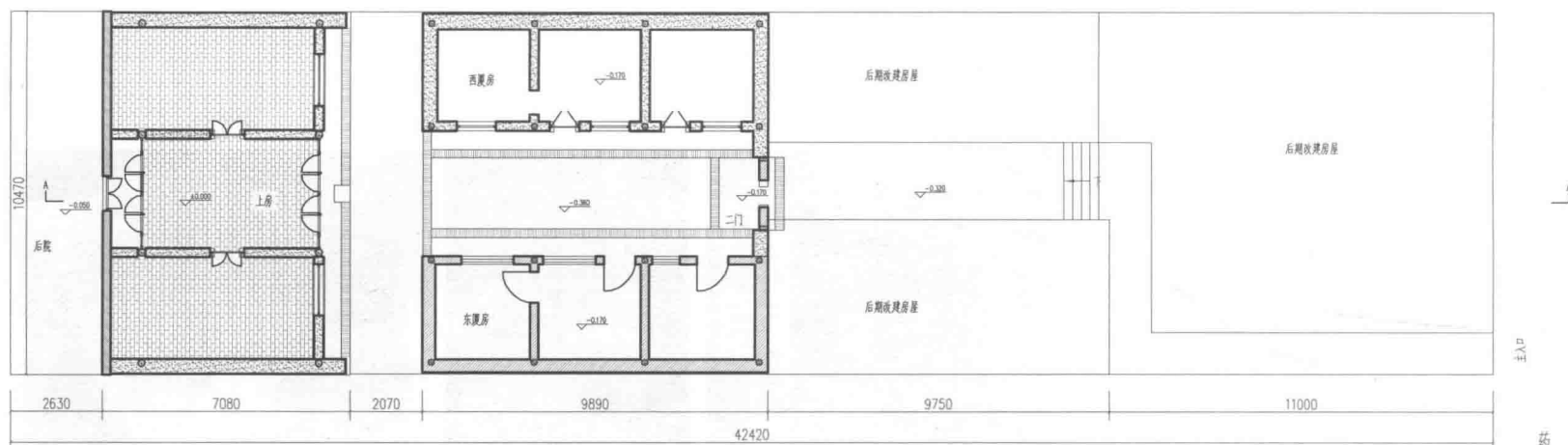
总平面图
