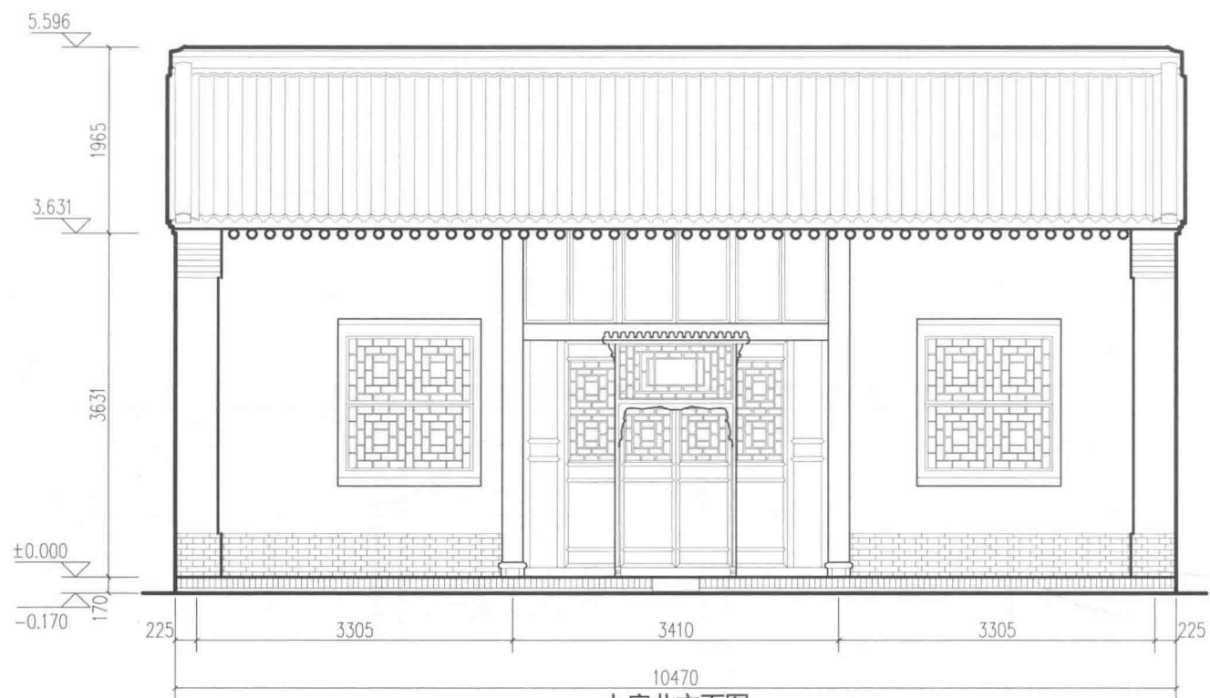
上房北立面图
