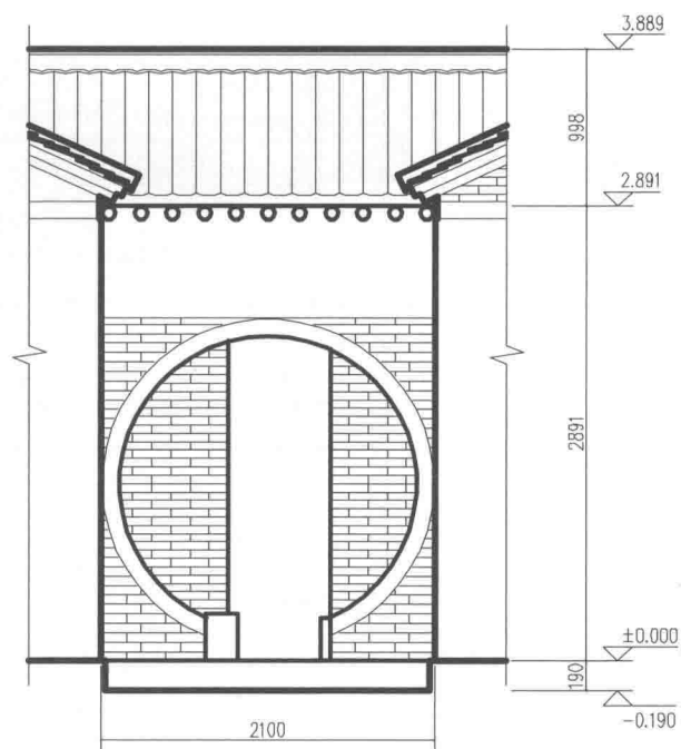
二门南立面图
