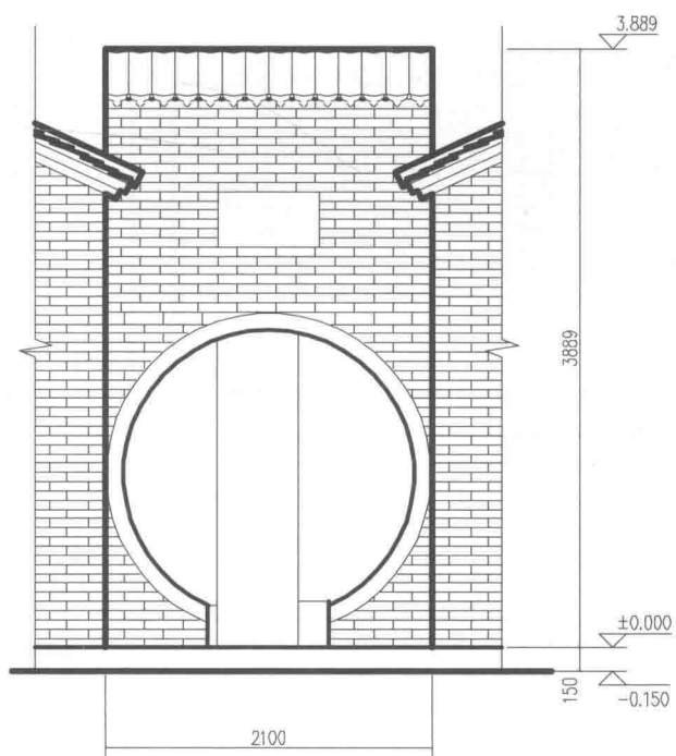
二门北立面图
