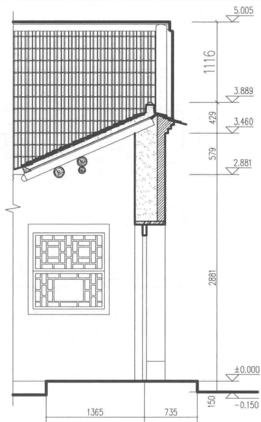
二门 2-2 剖面图
