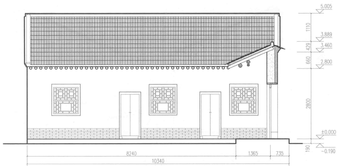
西厦房东立面图
