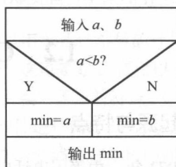
图 1.5 例 1.2 算法
