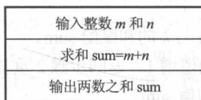
图 1.3 例 1.1 算法
