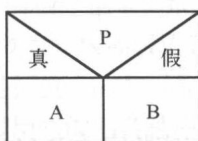
图 1.4 选择结构
