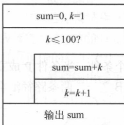
图 1.8 例 1.3 算法
