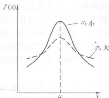
图 2.2-1 正态分布曲线
