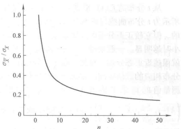
图 2.2-2 \sigma_{\bar{X}}/\sigma_X 与 n 的关系
