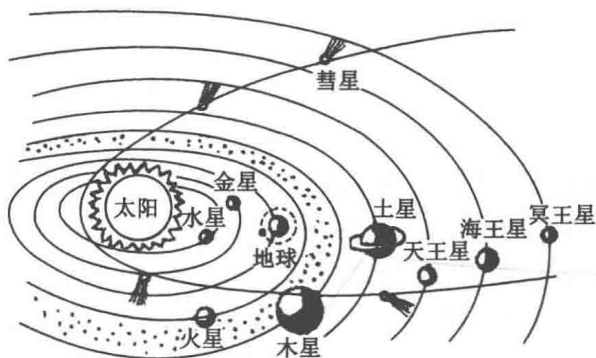
图 1.1 太阳系、地球在太阳系中的位置
