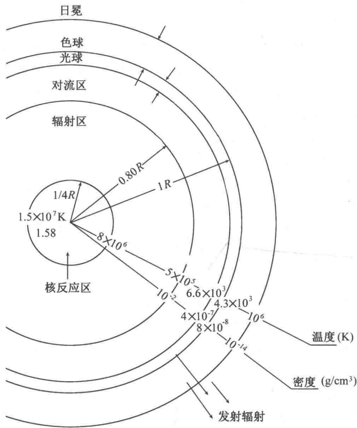
图 1.2 太阳结构示意图
