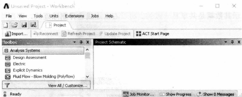
图 1-3 Workbench 界面
