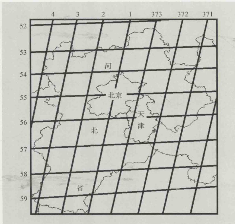
图 1-1 河北省CBERS影像覆盖示意图
