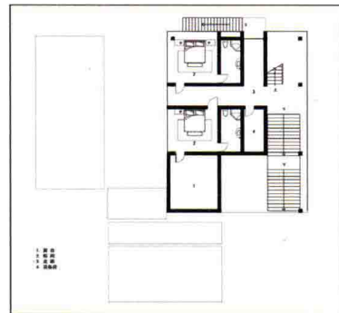
二层平面图 1: 100
