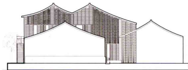
东南立面 1: 100
