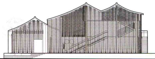
西北立面 1: 100
