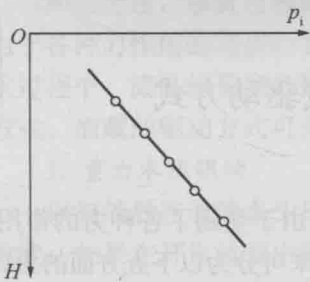
图 1-12 压力梯度曲线
