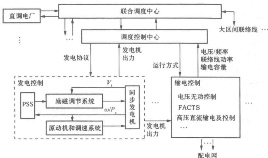
图 1-2 现代电力系统控制示意图
