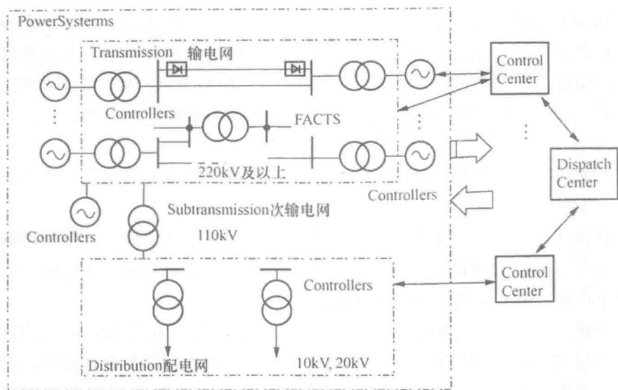
图 1-1 现代电力系统基本构成示意图
