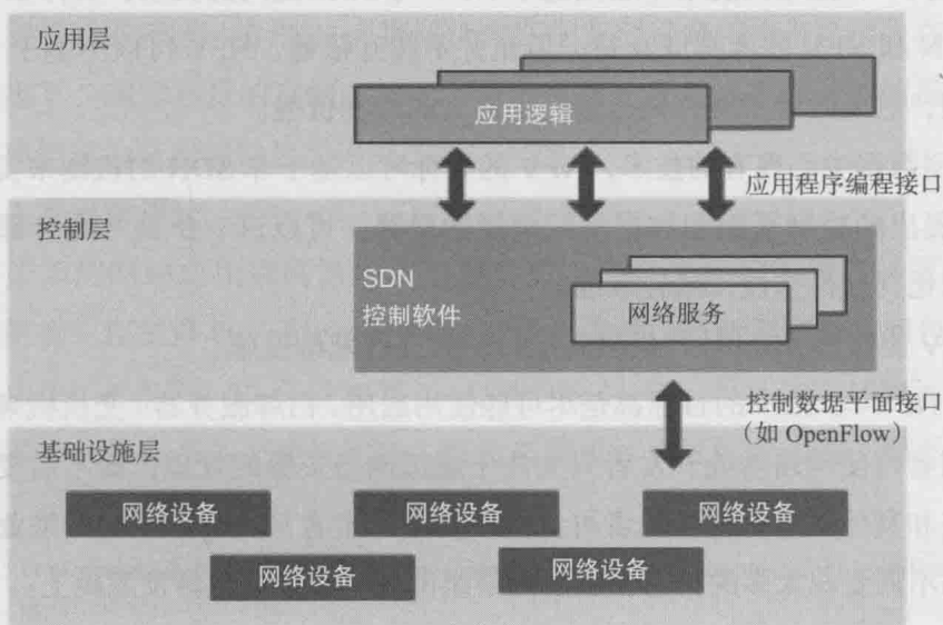
图 1-2 SDN 架构概览
