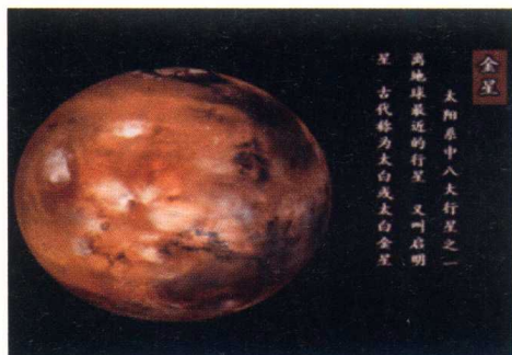
图 12 金星
