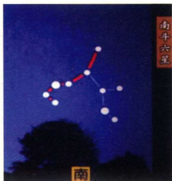
图11 南斗六星
