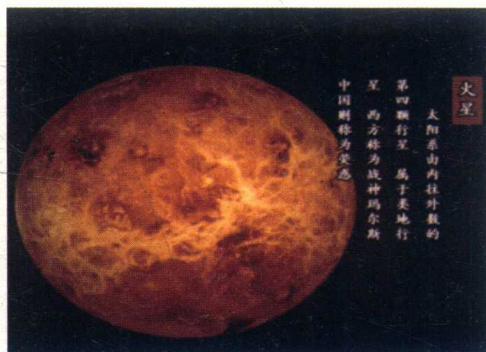
图 15 火星
