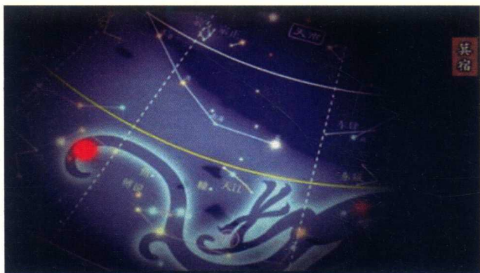
图7 箕宿（东方七宿末宿）
