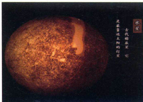
图 14 水星
