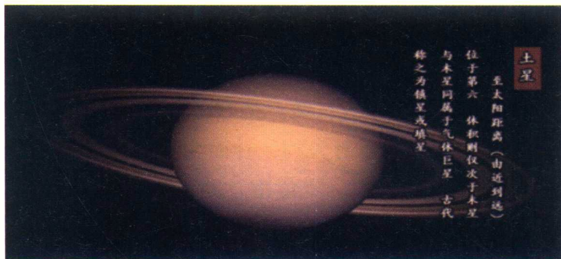
图 16 土星
