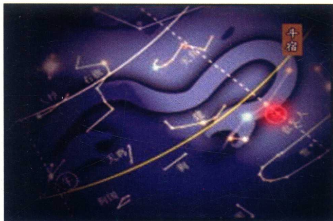
图8 斗宿（北方七宿第一宿）
