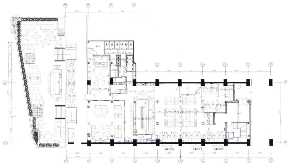
一层平面布置图
