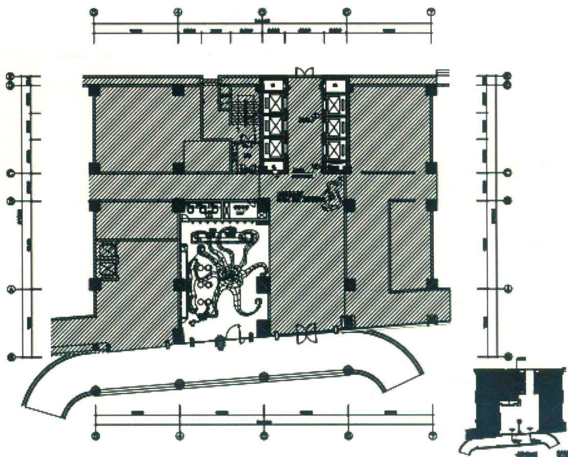
一层平面图
