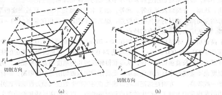
图 1-5 二维、三维切削与切削力
