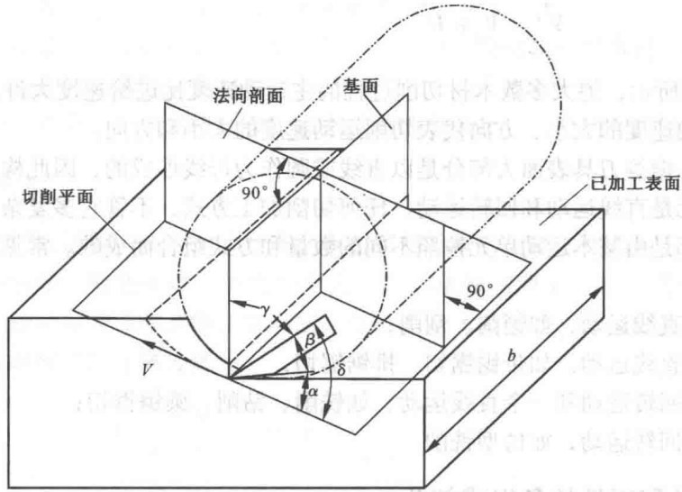
图 1-3 回转运动刀具的角度
