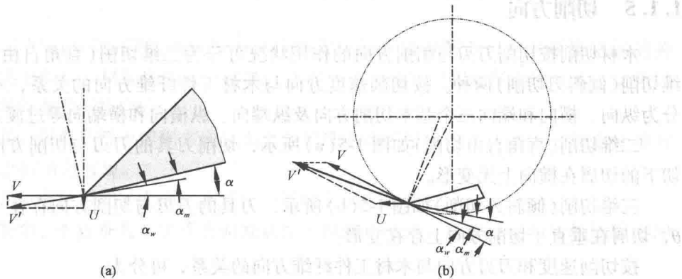
图 1-4 刀具后角和标注后角的关系
