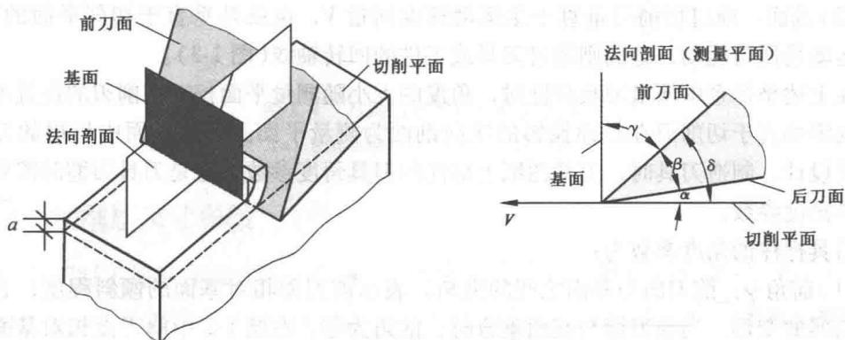
图 1-2 直线运动的刀具组成部分和角度
