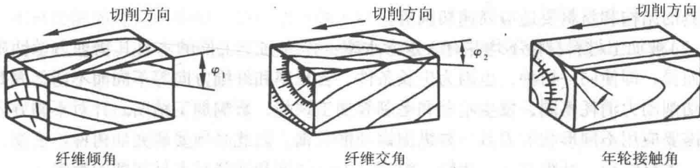
图 1-6 切削方向与木材工件纤维方向之间的角度关系
