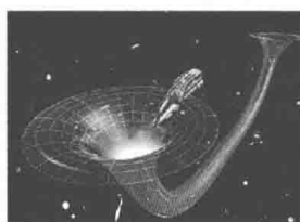
1-007 量子力学的表达※1
