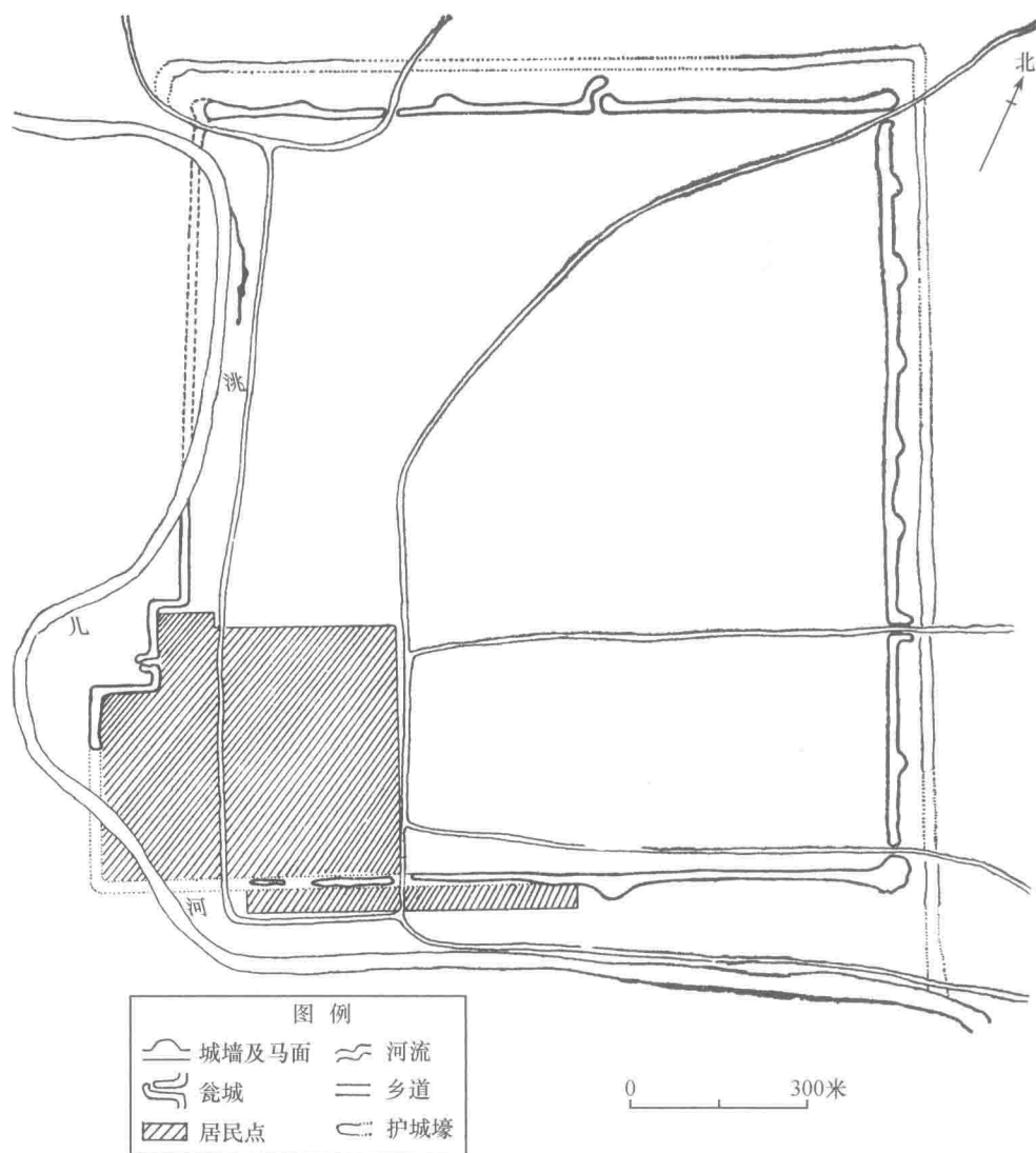
图二六六 城四家子古城平面图
