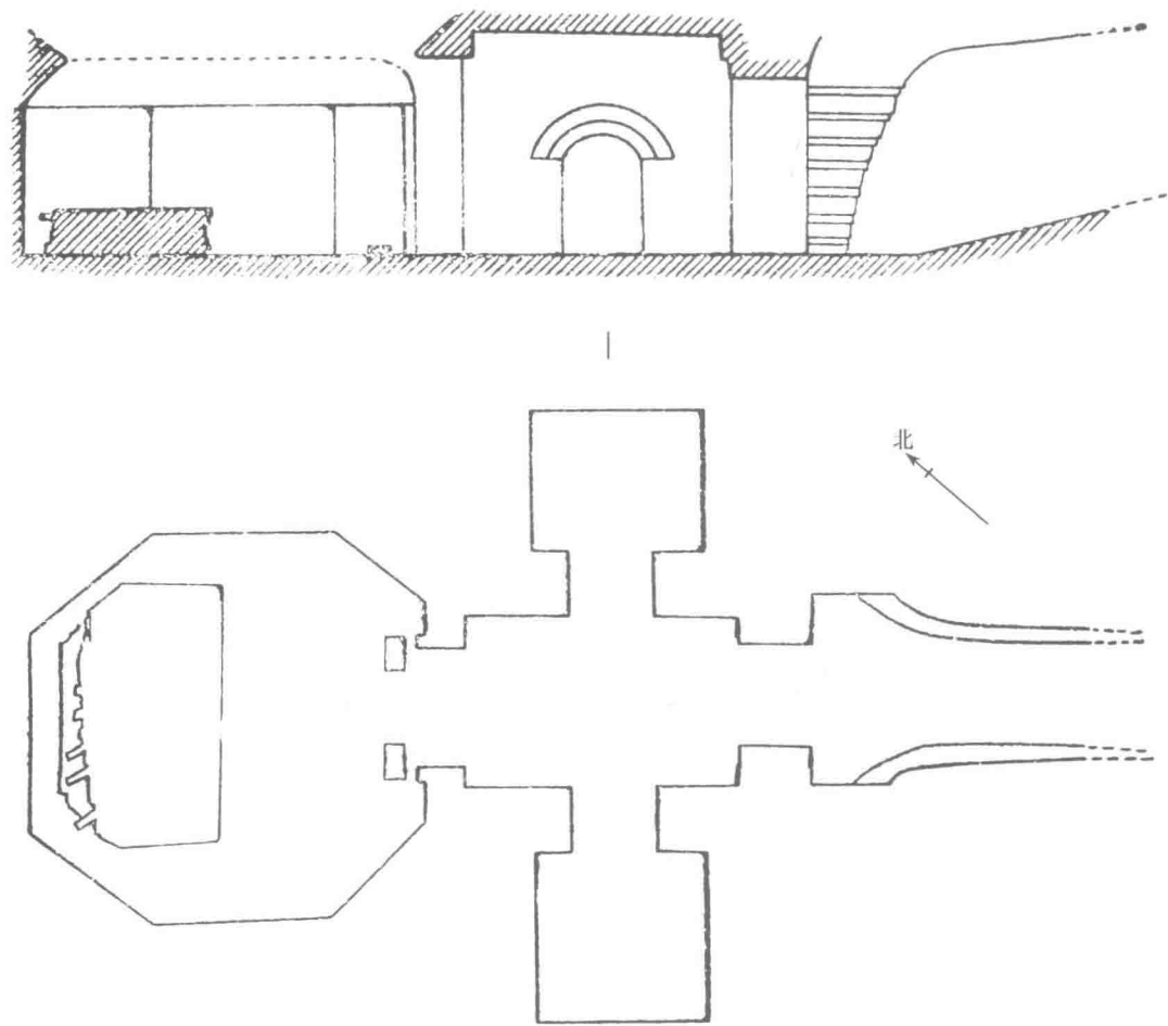
图二七三 双辽骆驼岭辽墓平、剖面图
