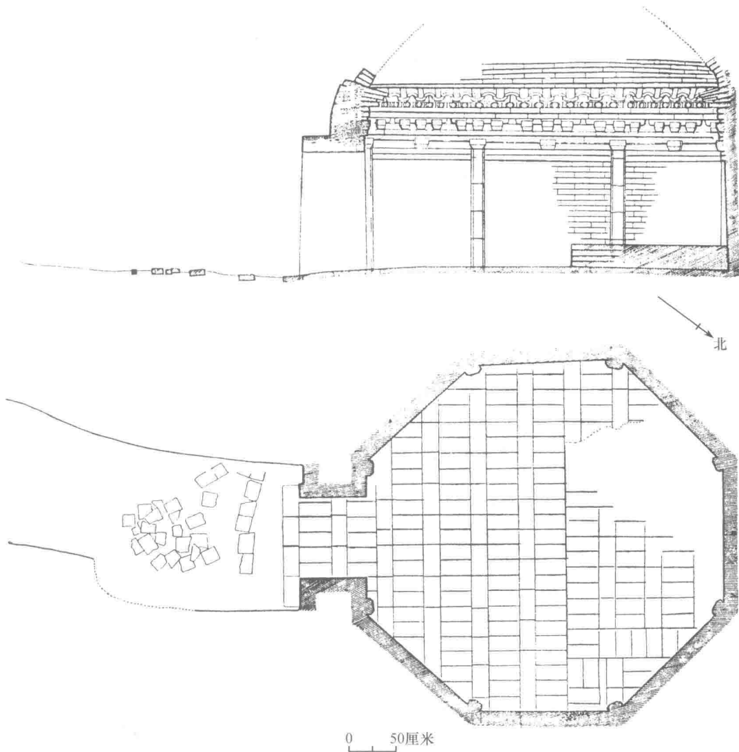
图二七二 梨树胡家屯M1平、剖面图
