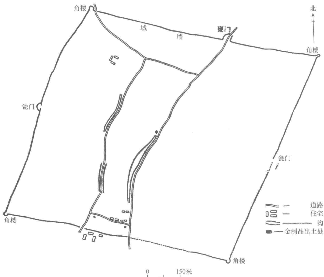
图二六八 梨树偏脸城平面图
