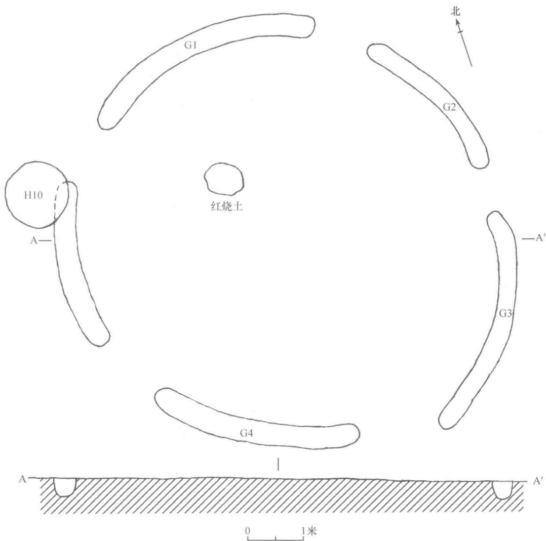
图二七〇 双辽后太平遗址I区F1平、剖面图
