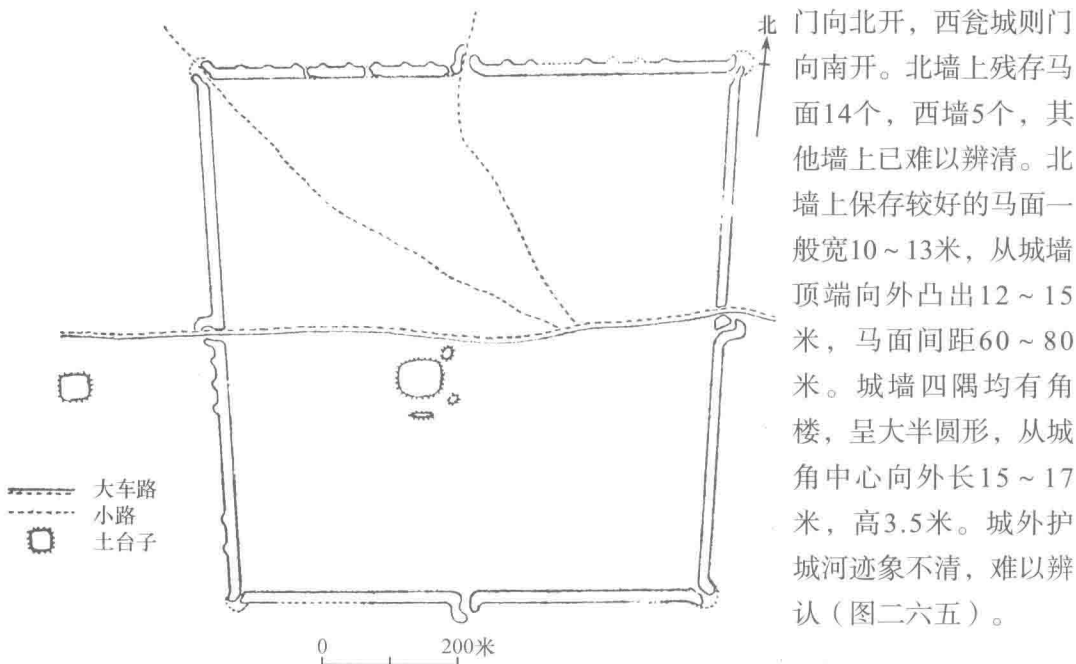
图二六五 伯都古城平面图
