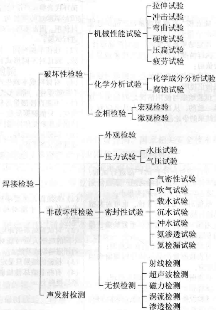
图 1-1 常用焊接检验方法
