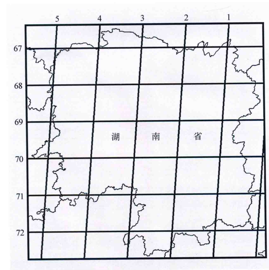
图 1-1 湖南省CBERS影像覆盖示意图
