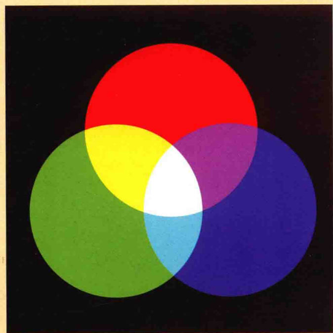
◆图 4-43 三原色
