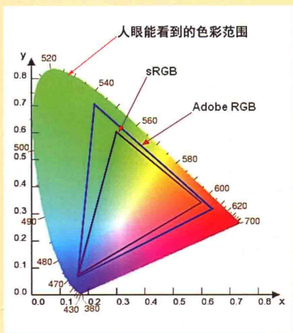
◆图 3-72 色彩空间
