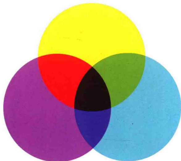
◆图 4-44 三补色
