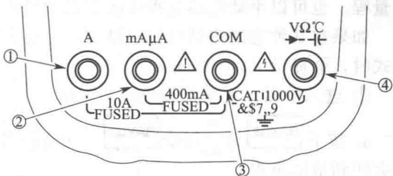
图 1. 2. 4 Fluke 17B 型数字万用表的外接端子
