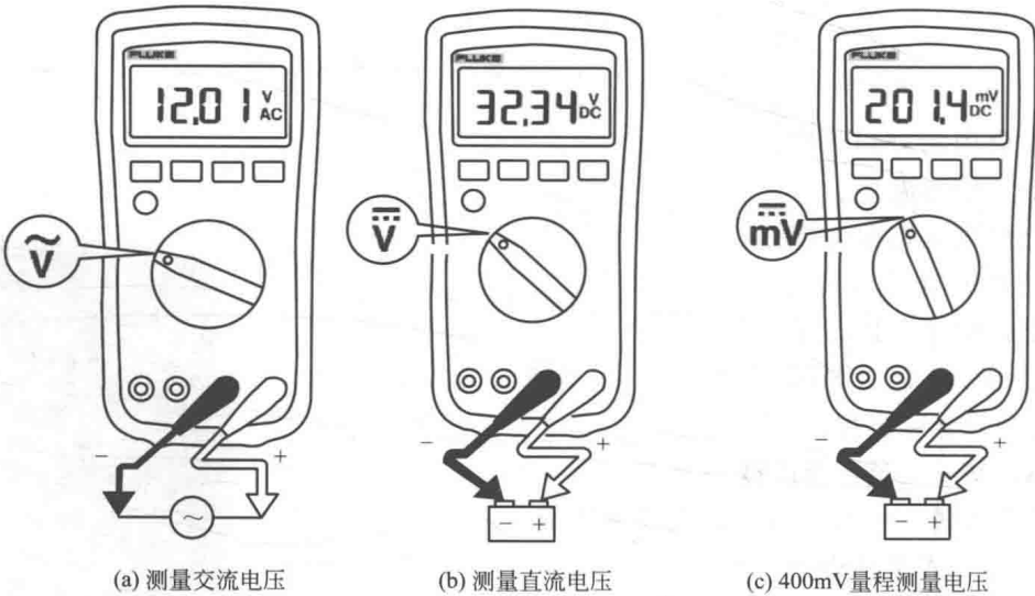
图 1.2.6 测量交流和直流电压
