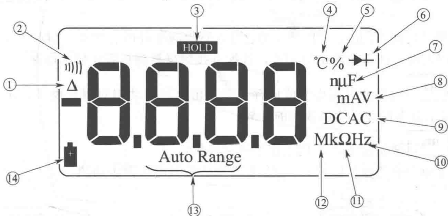
图 1. 2. 5 Fluke 17B 型数字万用表的显示屏
