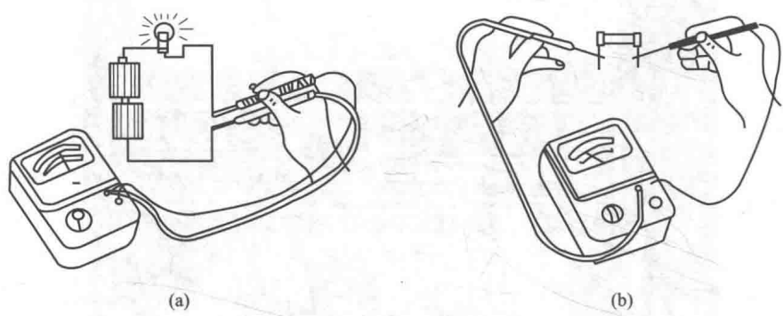
图 1.2.2 万用表表笔的握法
