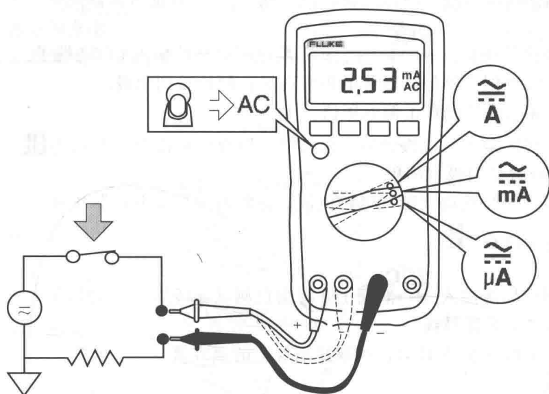
图 1.2.7 测量交流和直流电流
