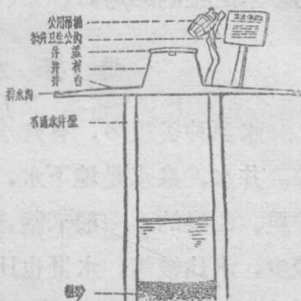
图一 标准井
