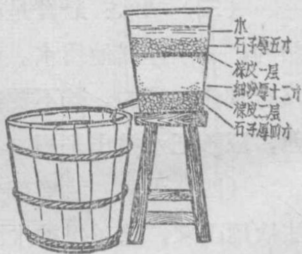
图三 沙滤桶
