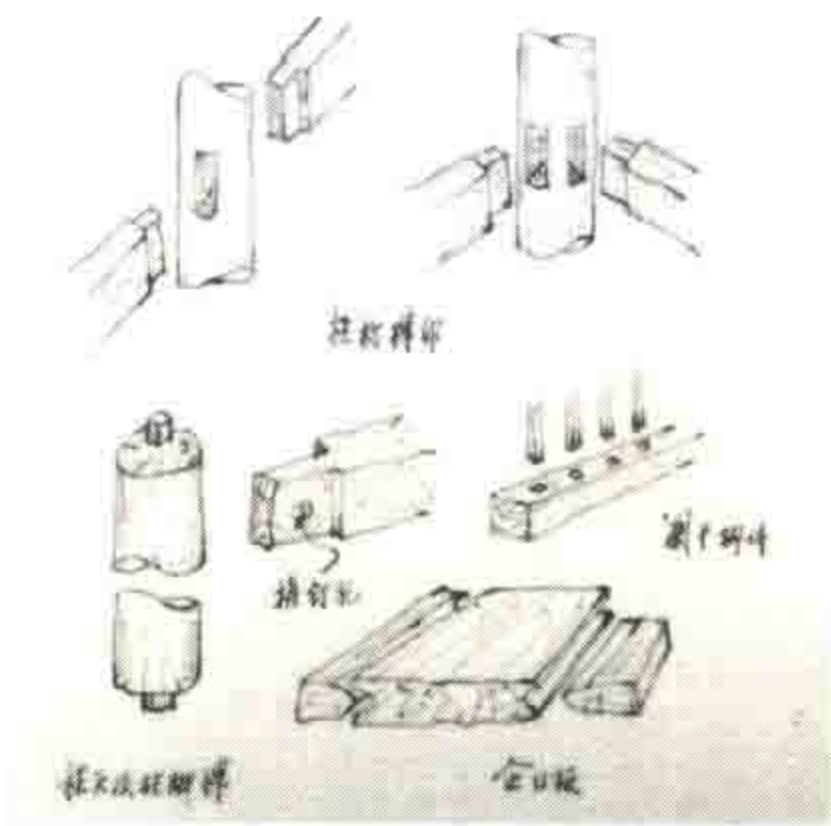
河姆渡遗址房屋榫卯
