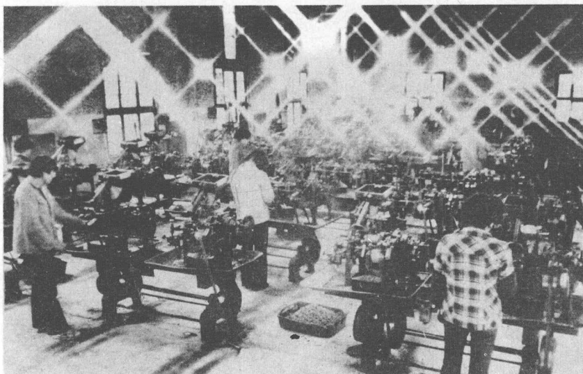
◁海盐螺丝厂螺纹车间一角
