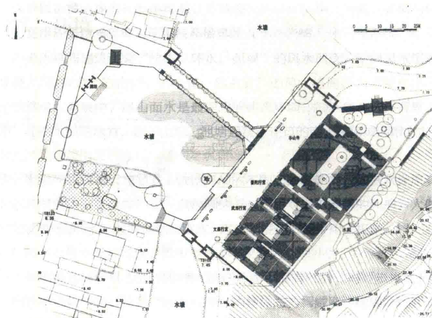
图 2-4 胥江祖庙总平面图
