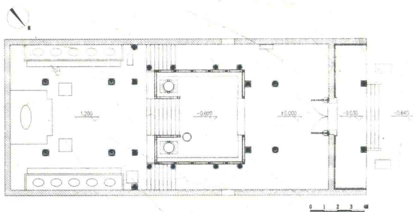
图 2-5 胥江祖庙武当行宫平面图
