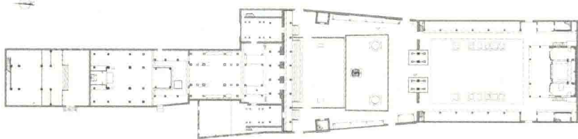
图 2-2 佛山祖庙庆真楼（左）、灵应祠、锦香池、灵应牌坊、万福台（右）平面图 图片来源：佛山市祖庙博物馆提供
