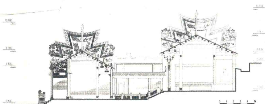
图 2-6 胥江祖庙武当行宫横剖面图
