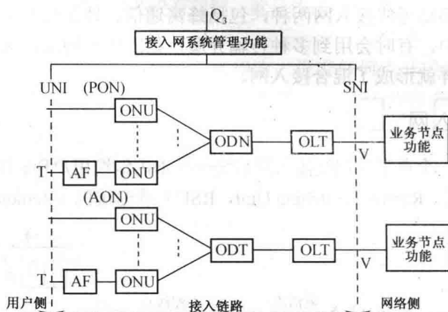
ONU: 光网络单元 PON: 无源光网络 UNI: 用户网络接口 ODN: 光配线网络 OLT: 光线路终端 AON: 有源光网络 SNI: 业务节点接口 T: T接口 AF: 适配功能 ODT: 光配线终端 V: V接口 Q 3 : Q 3 接口
