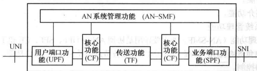
图 1-4 接入网功能结构
