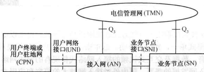
图 1-2 接入网的定义
