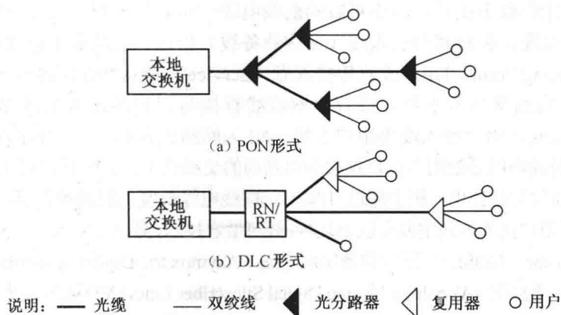
图 1-9 树型—分支结构
