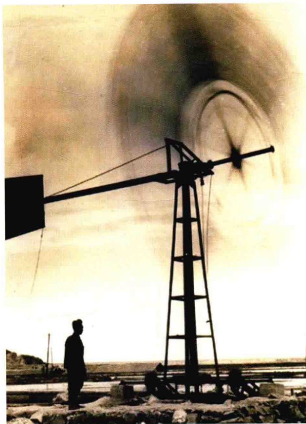
图版 47-004-4 20 世纪 60 年代盐场风车带螺旋泵扬水 (《宁波盐志》，宁波出版社 2009 年版，图版第 13 页)
