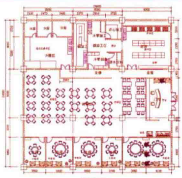
餐厅装饰平面图
