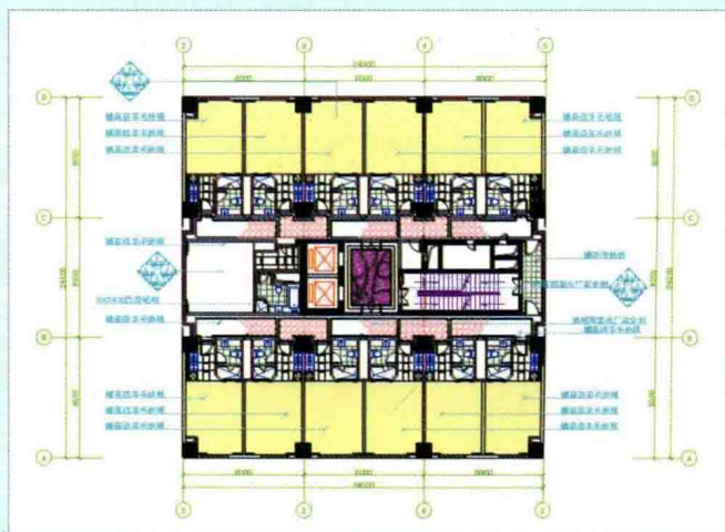
■ 十八层地坪图的绘制
