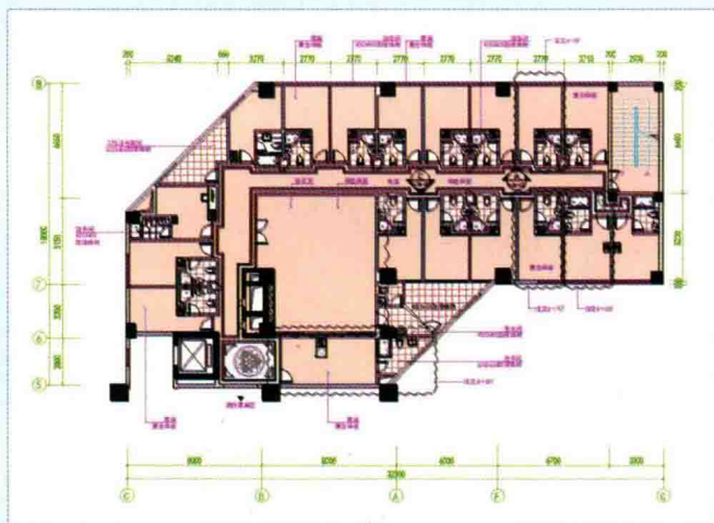
■ 十六七层地坪图的绘制
