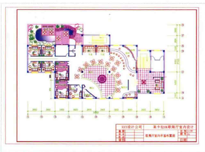
歌舞厅室内平面图
