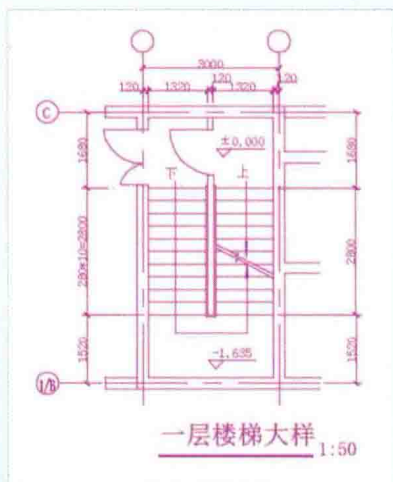
楼梯大样图
