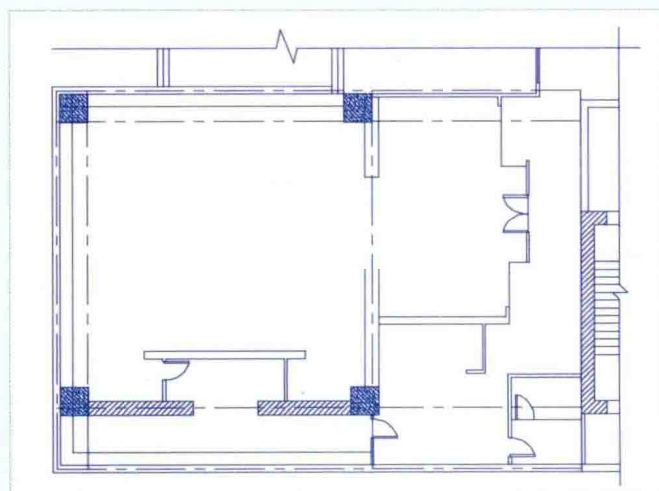
■ 董事长室平面图
