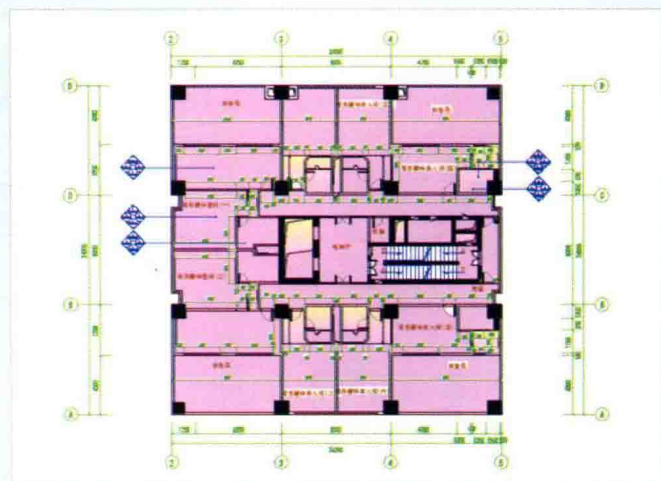
十九层客房平面图
