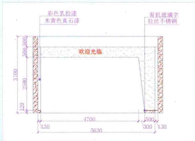
一层过道处隔断立面
