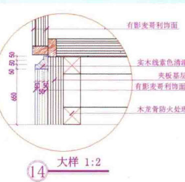
绘制节点大样图13
