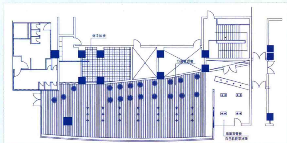
■ 咖啡吧顶棚图
