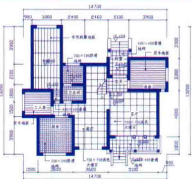
别墅首层地坪图的绘制
