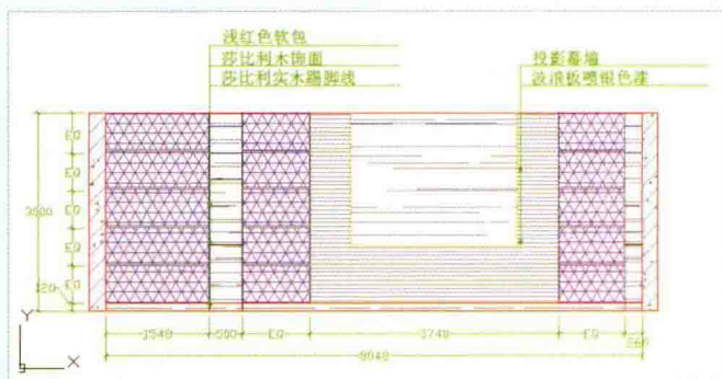
会议室投影墙面装饰立面
