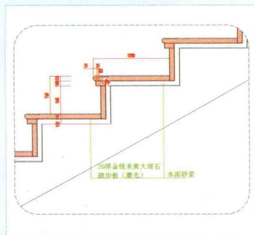
■ 踏步大样图的绘制
