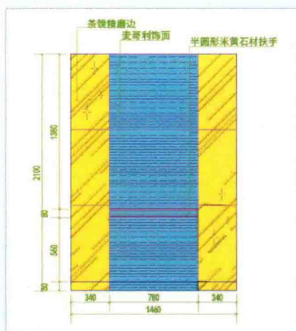
■ 电梯右侧立面图
