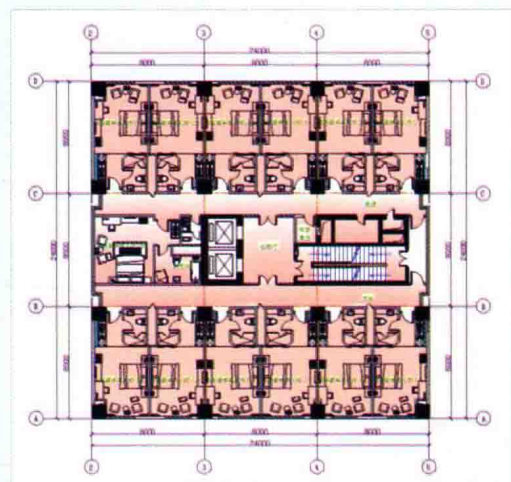
十八层装饰平面图
