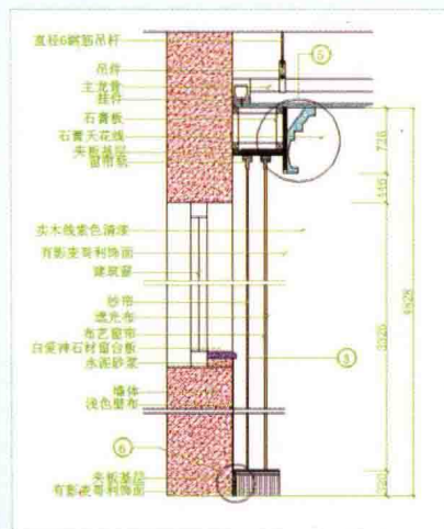
4. 单人间剖面图的绘制
