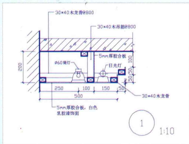
住宅室内吊顶构造详图
