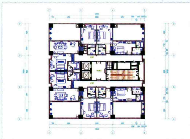
■ 十九层装饰平面图
