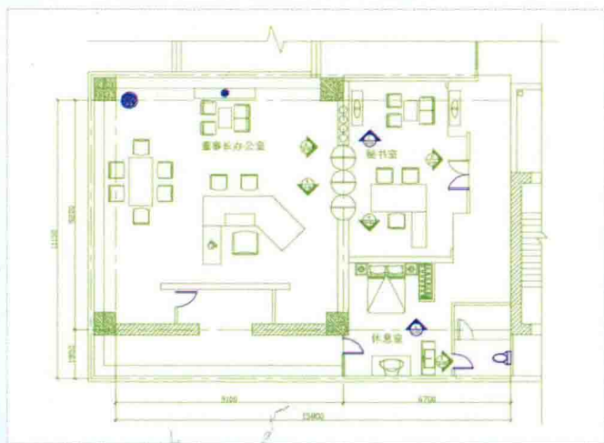
董事长室装饰平面图
