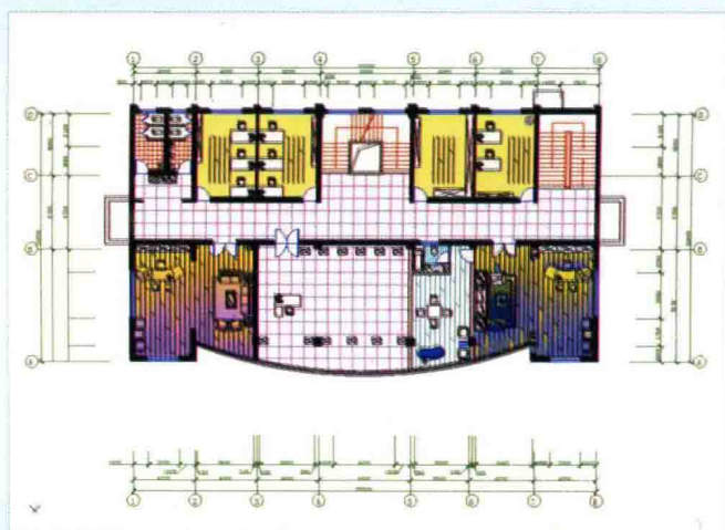
二层地坪图
