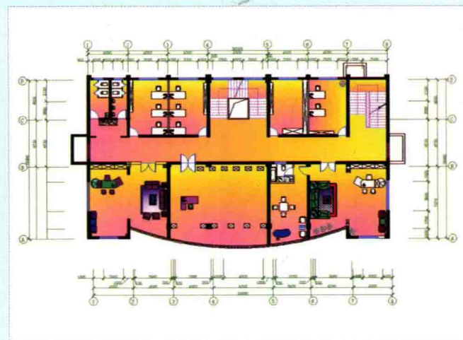
二层装饰平面图
