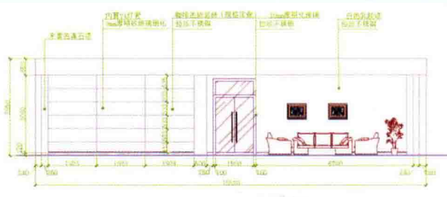
大厅背景墙立面
