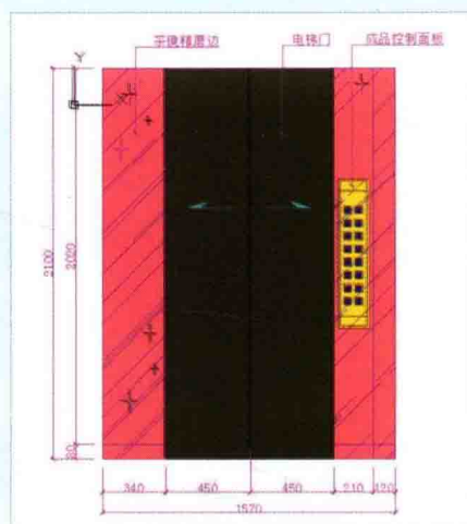
■ 电梯门立面图
