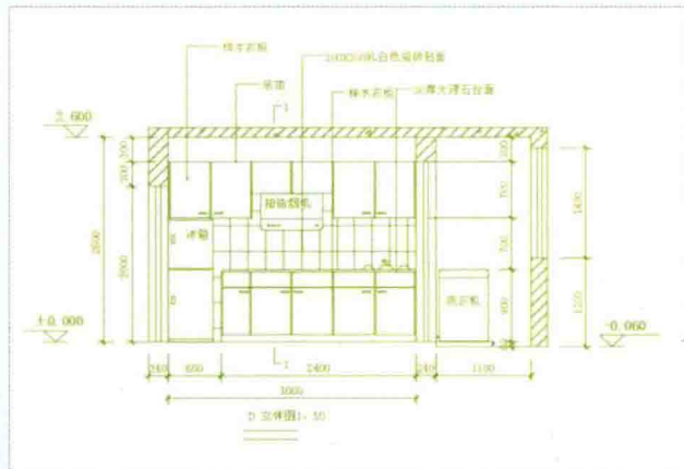
住宅室内D立面图
