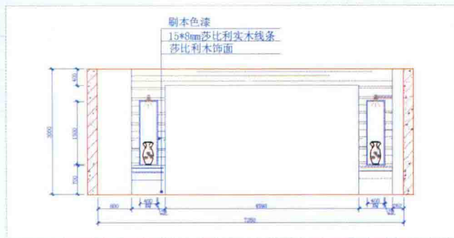
总经理室隔断立面
