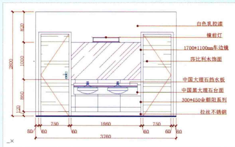
■ 一层卫生间台盆立面
