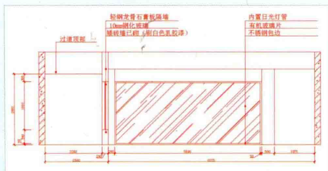
样品间展示墙立面
