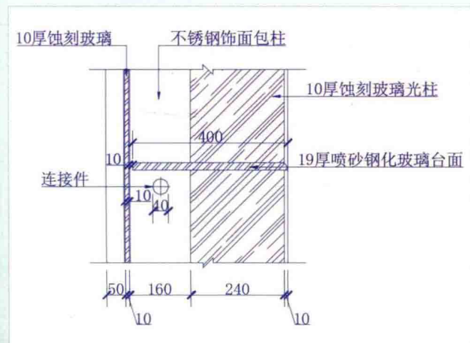
咖啡吧玻璃台面节点详图
