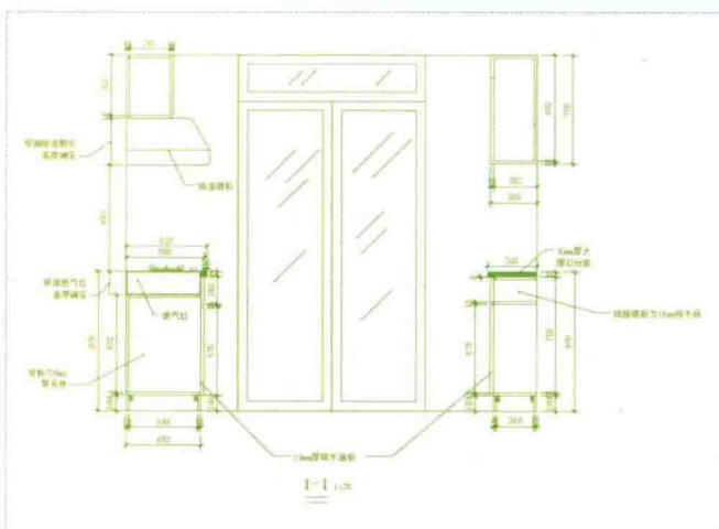
住宅室内家具详图
