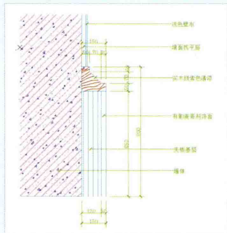
■ 绘制节点大样图6
