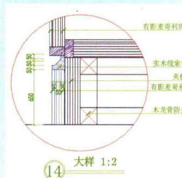
绘制节点大样图14
