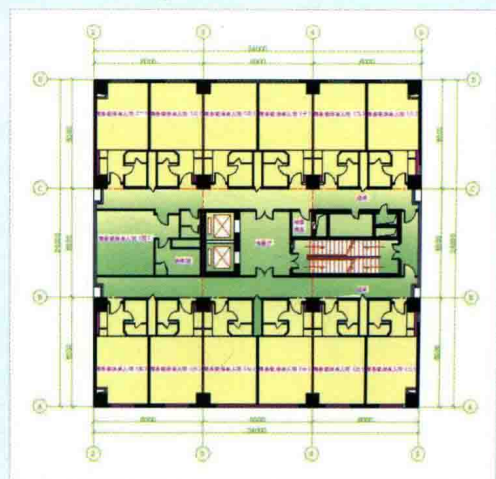
■ 十八层客房平面图
