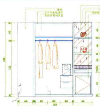
单人间衣柜开启立面图
