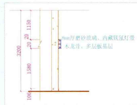
大厅背景墙剖面图的绘制
