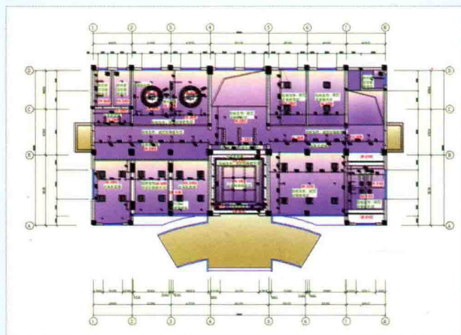
■ 一层顶棚平面图
