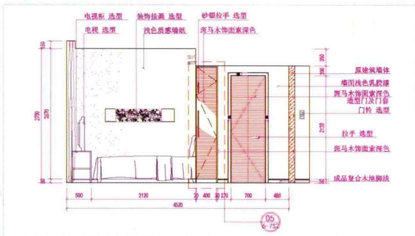
客房7卧室立面图
