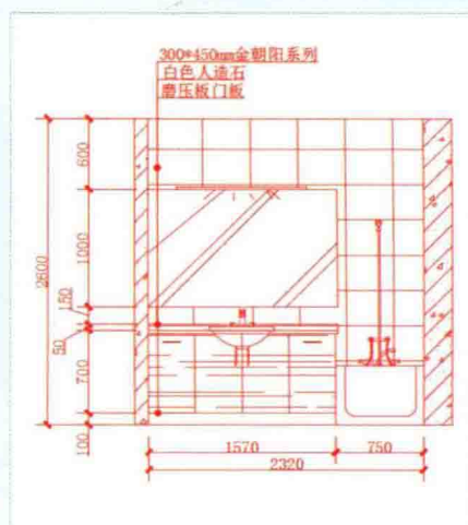
包间卫生间墙面装饰立面
