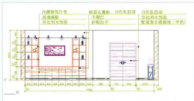
总经理室资料柜立面
