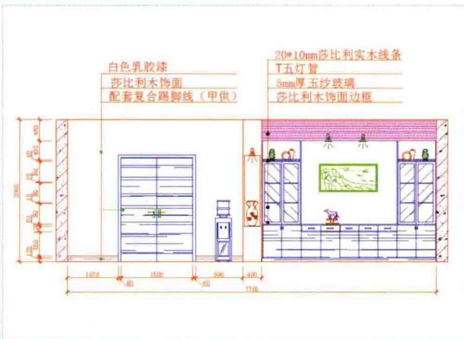
董事长室资料柜立面
