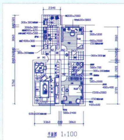
住宅装饰平面图
