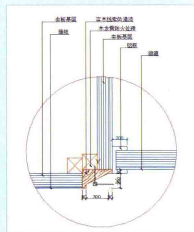
■ 绘制节点大样图
