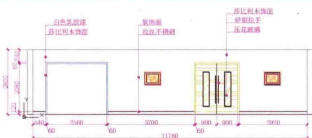
过道客人餐厅大门立面
