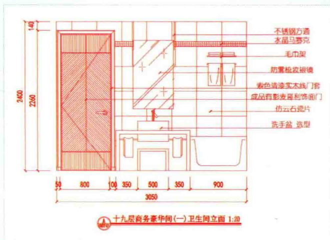
■ 商务豪华套间卫生间立面图
