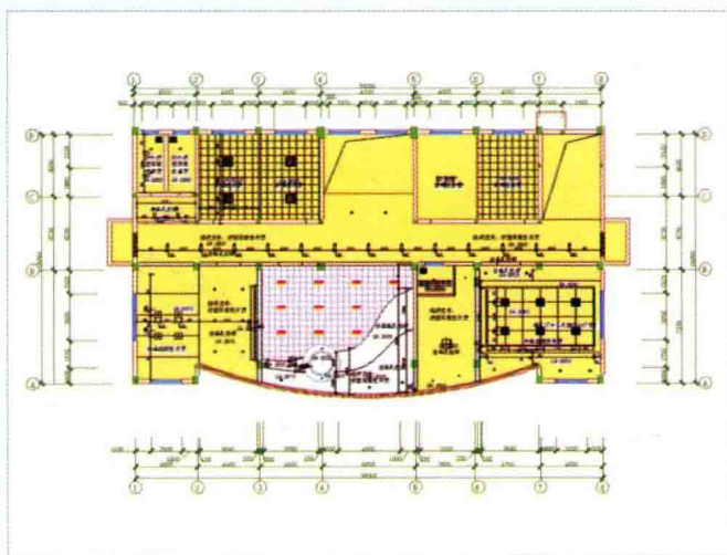
二层顶棚平面图
