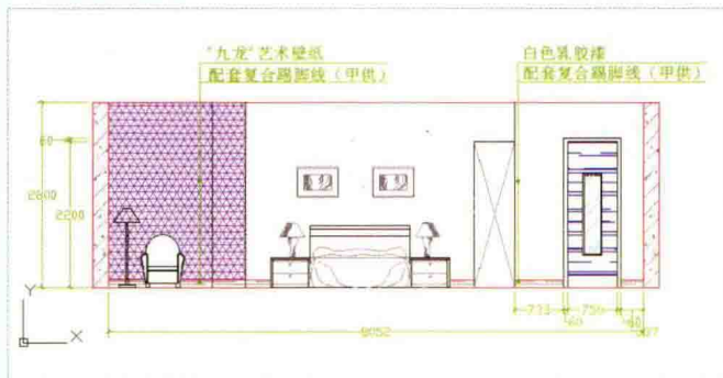
客房包间墙面装饰立面
