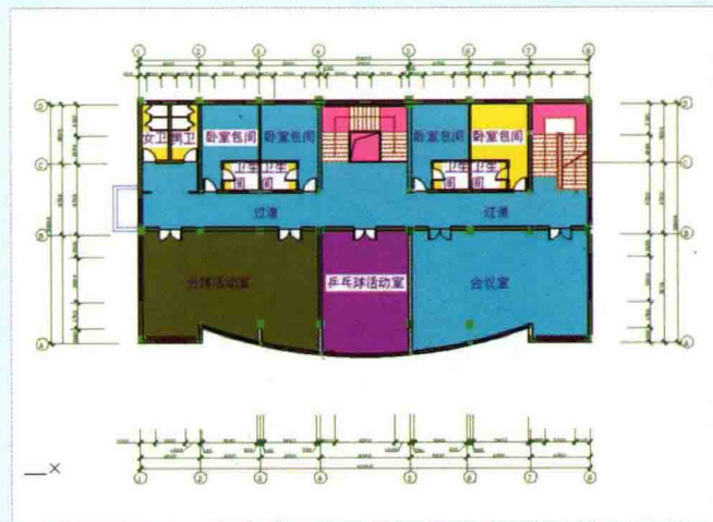
三层平面图
