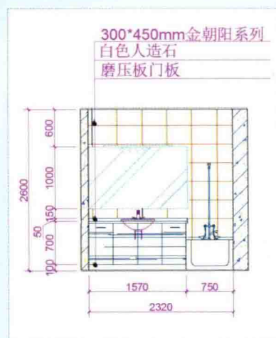
■ 休息室卫生间墙面立面
