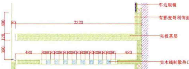
绘制节点大样图16
