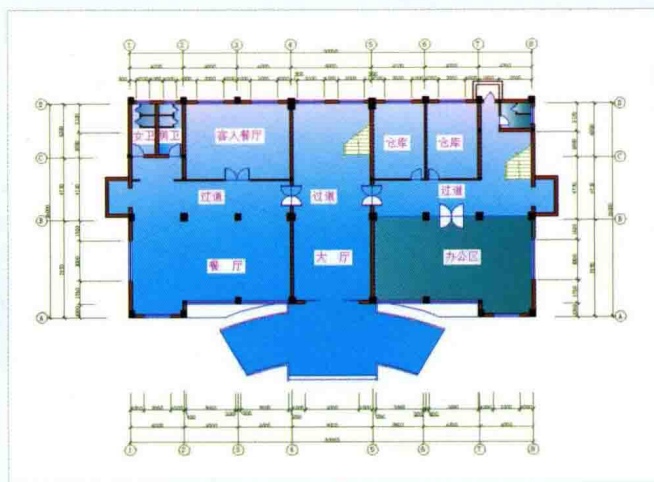
一层平面图
