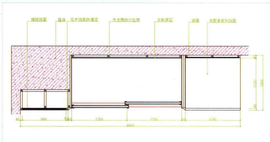
十八层商务豪华单人间衣柜剖面图的绘制
