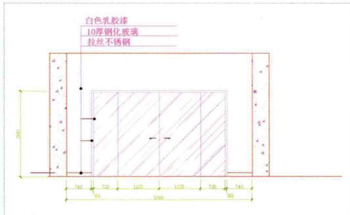
大厅感应大门立面图
