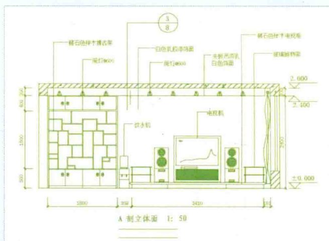
住宅室内A立面图
