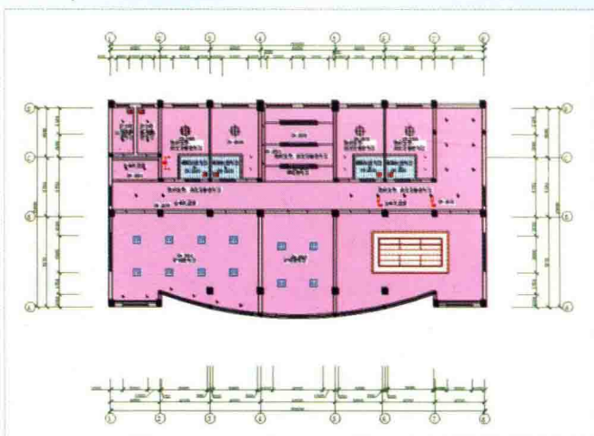
三层顶棚平面图
