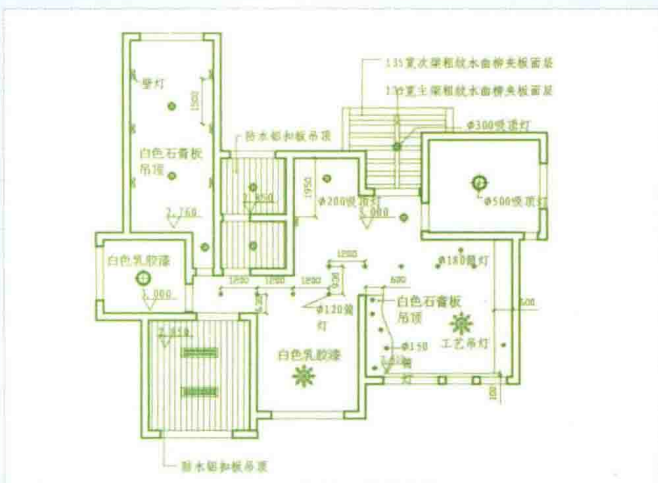
别墅首层顶棚图的绘制
