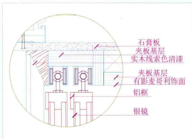
■ 绘制节点大样图11
