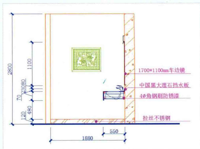
■ 卫生间台盆剖面图的绘制
