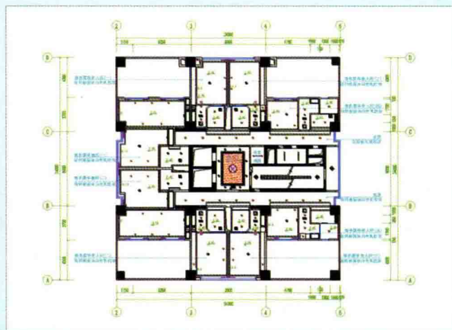
■ 客房地坪装饰图
