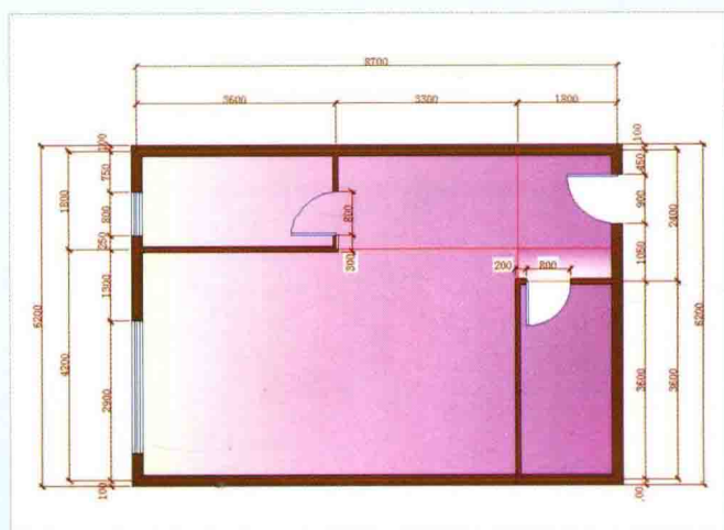
给居室平面图标注尺寸
