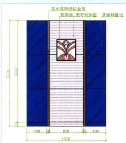
电梯门背立面图
