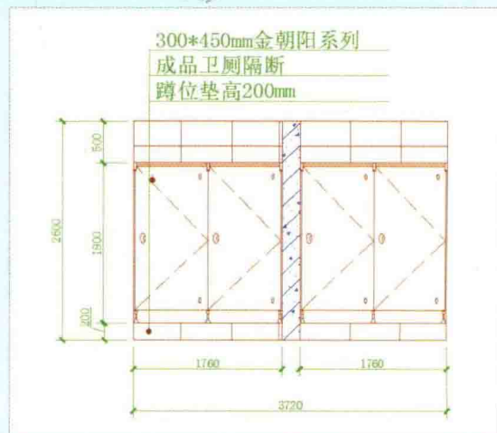
■ 成品卫厕所隔断立面
