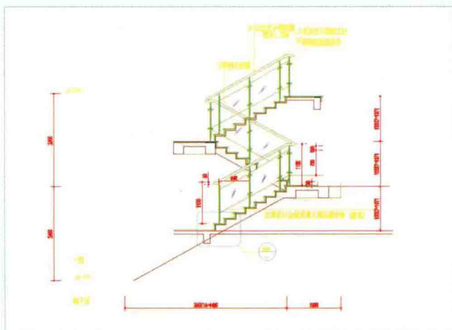
■ 主楼梯立面
