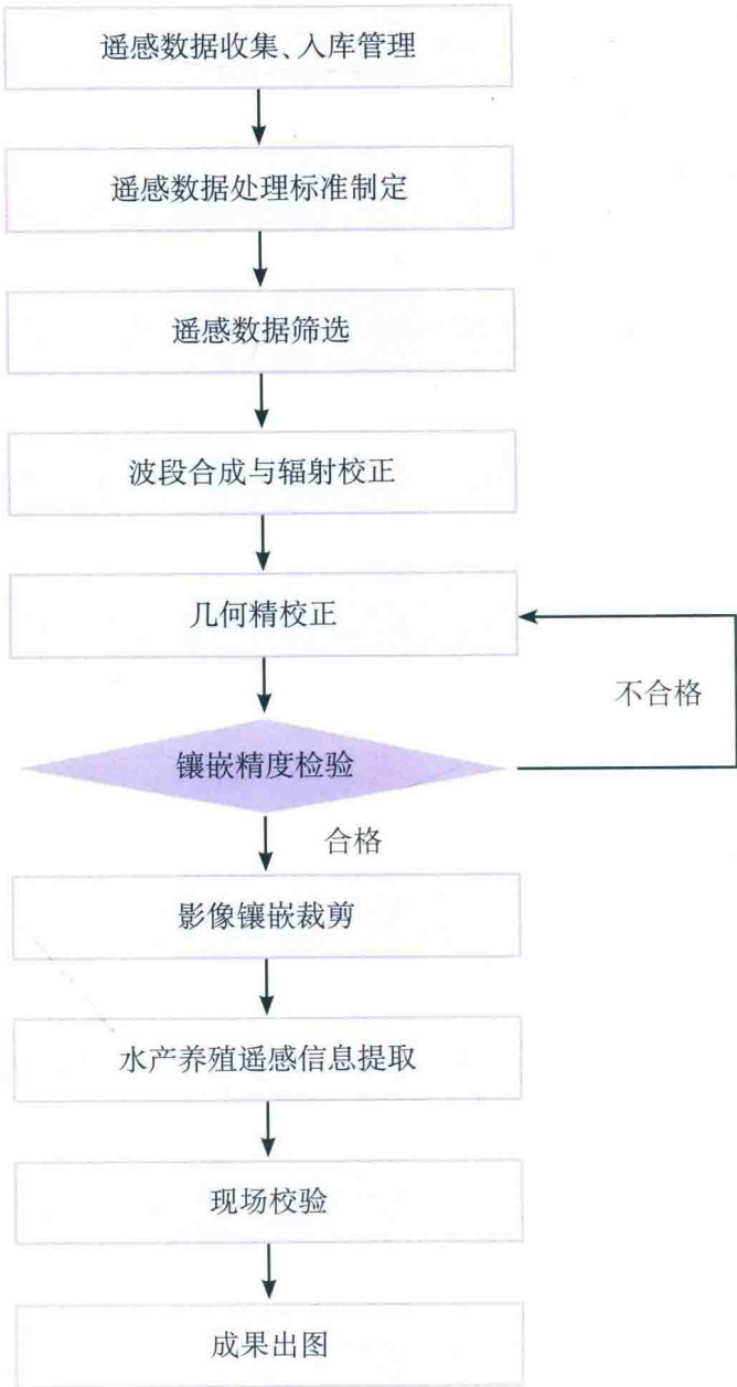
图 1-2 水产养殖水体资源遥感普查技术流程图
