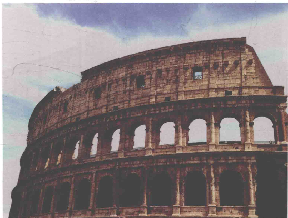
图 2.3 罗马竞技场
