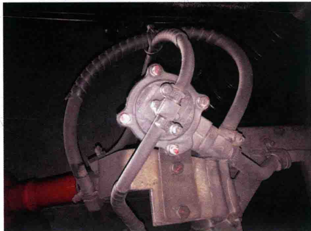
ADD 降弓阀
