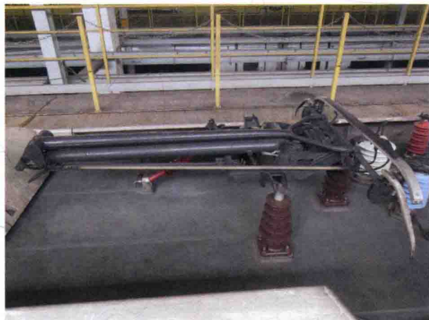
受电弓
