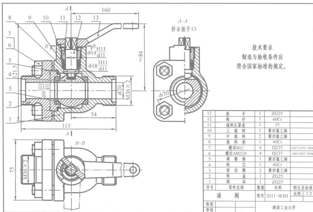
图 0-5 球阀装配图
