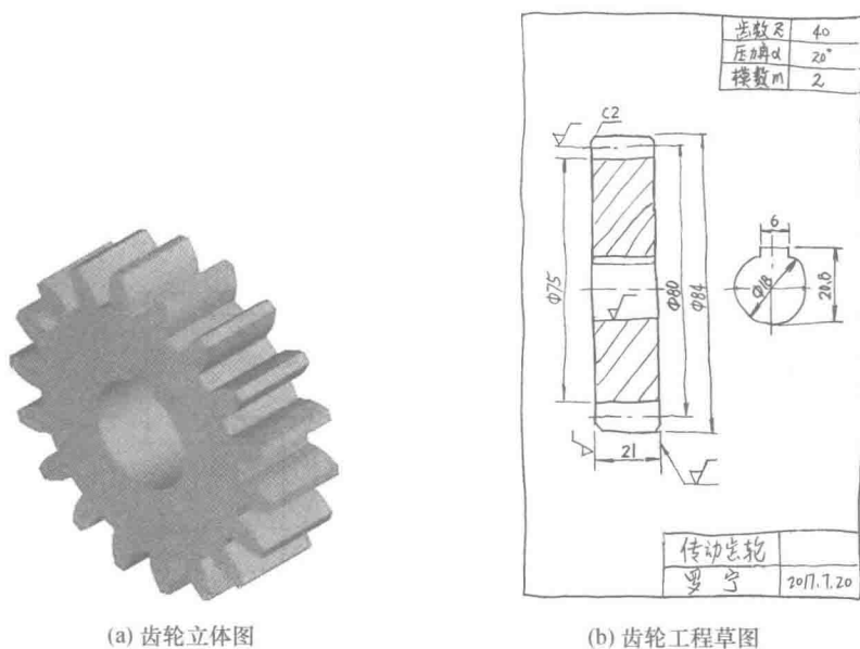
图0-19 齿轮立体图与工程草图
