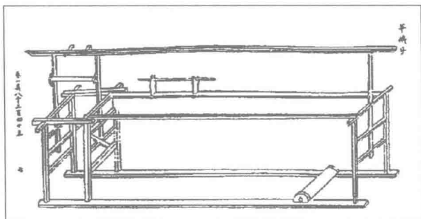
图 0-11 《梓人遗作》中的纺织机械图
