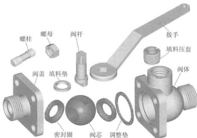
图 0-6 球阀分解图
