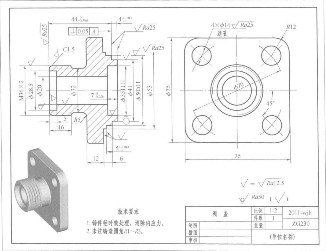
图 0-7 阀盖立体与阀盖零件图
