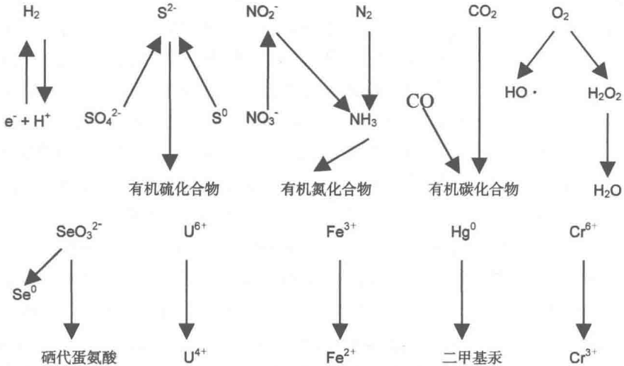
图 1-1 硫酸盐还原菌参与的化学转化过程
