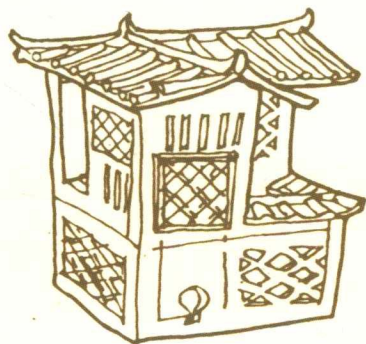
干栏式住宅
