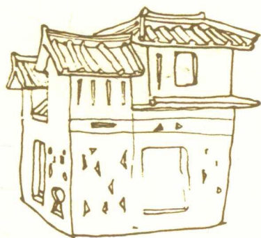
干栏式住宅
