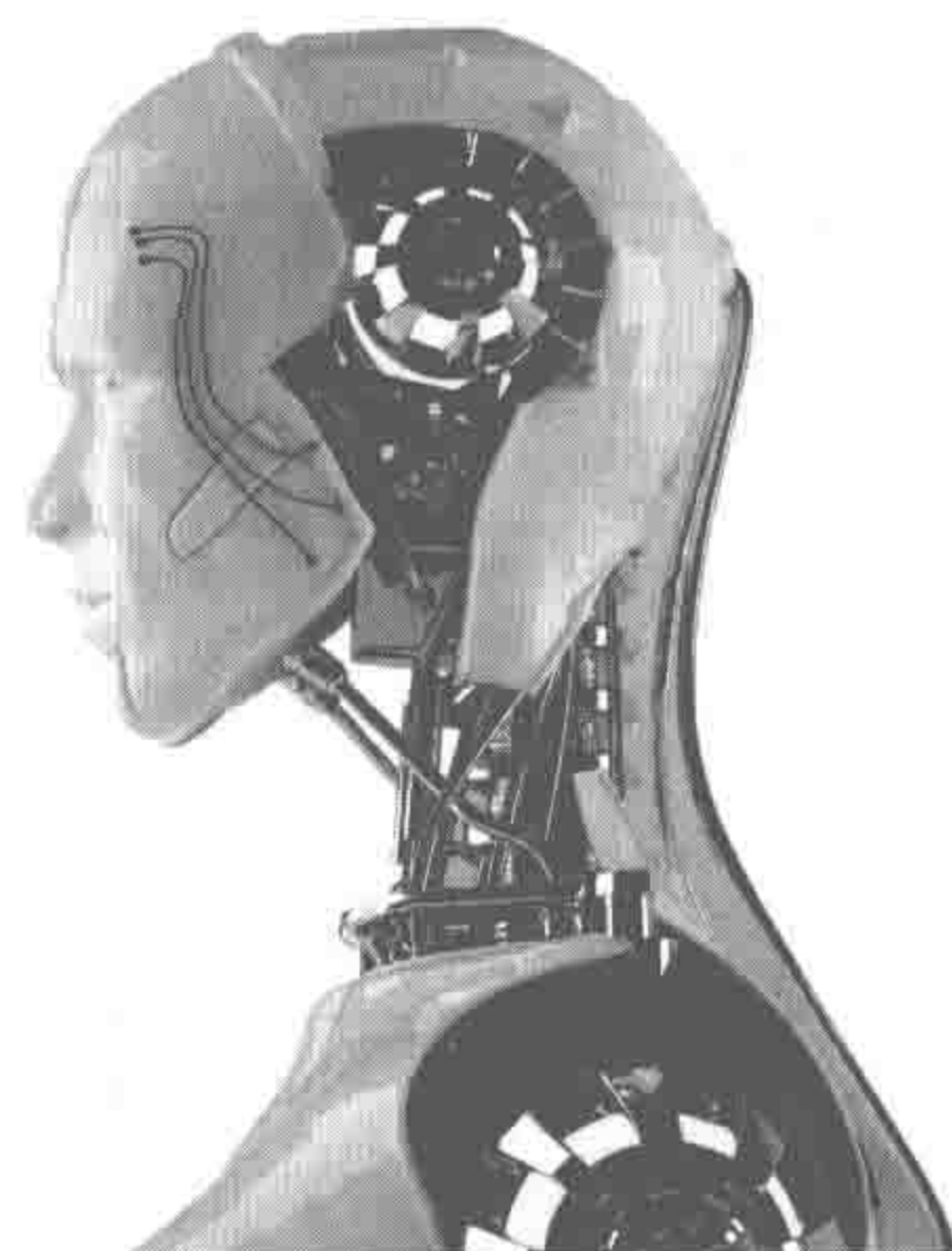
白方：（Master）AlphaGo
