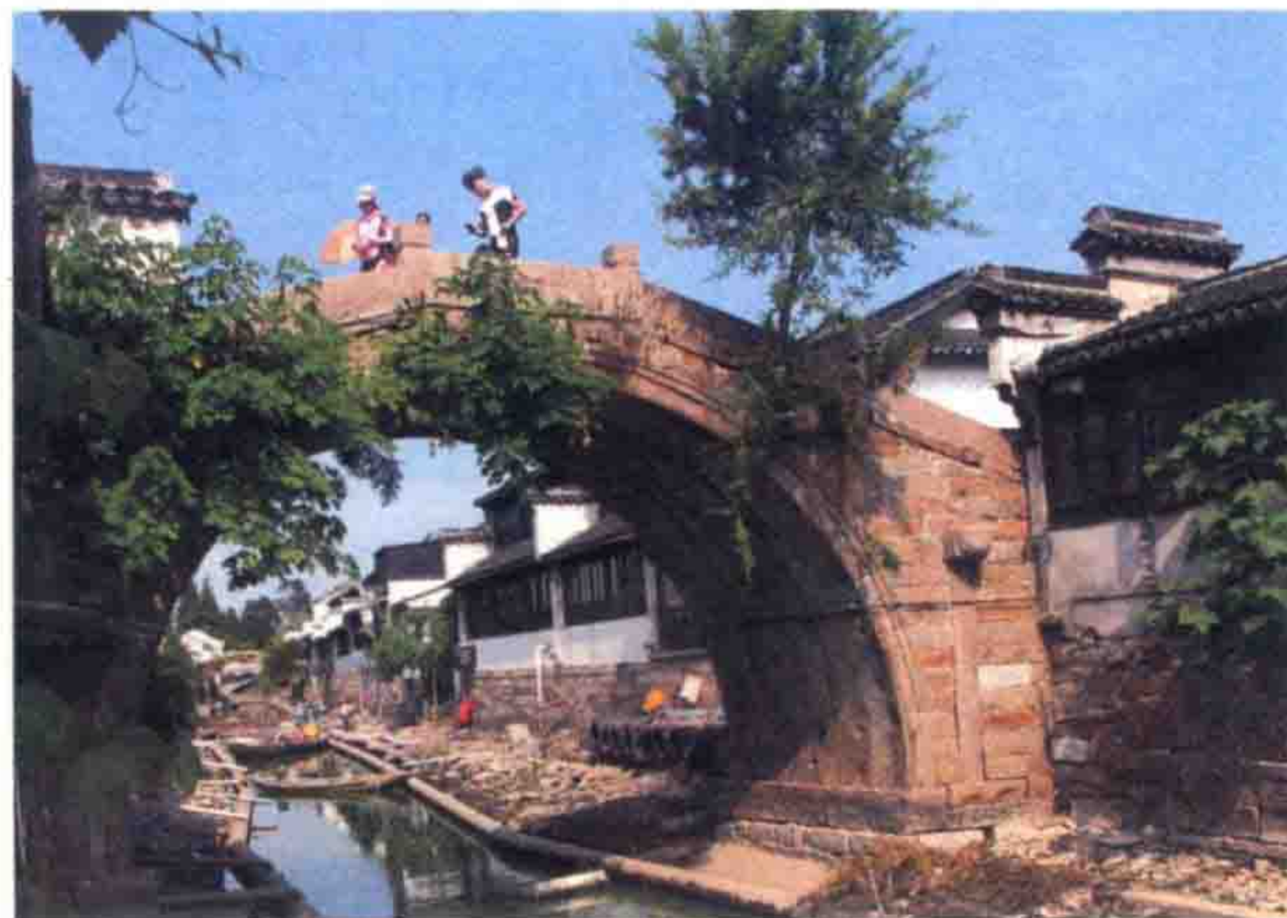
江苏省太仓市沙溪镇庵桥
