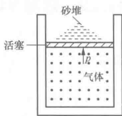
图 11-2 准静态过程
