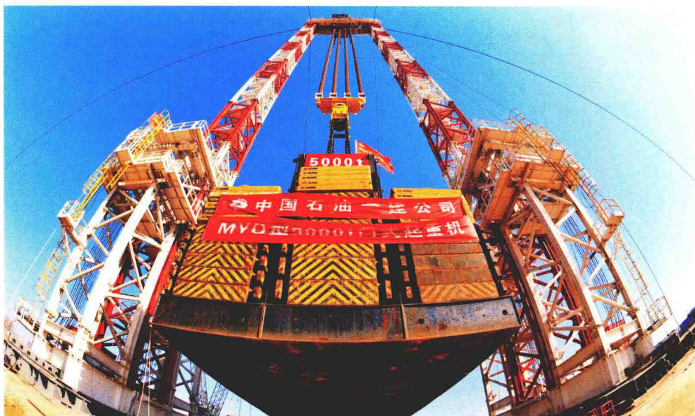
中国石油一建研发制造的 MYQ 型 5000 吨门式起重机
