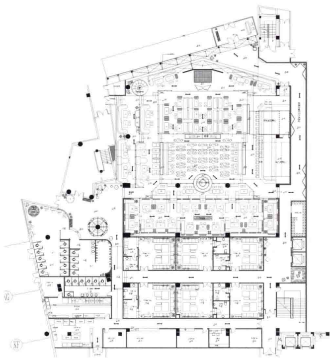
平面布置图
