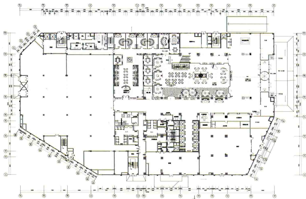
一层平面布置图
