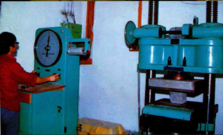
公路总段拌合厂压力试验
