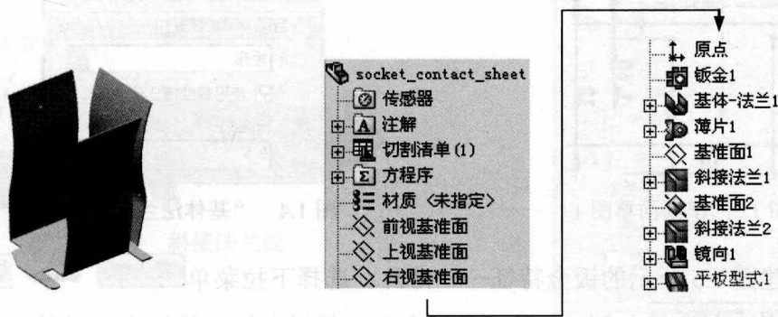
图 1.1 钣金件模型及设计树
