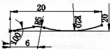
图 1.11 横断面草图 3
