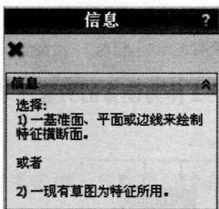
图 1.9 “信息”对话框
