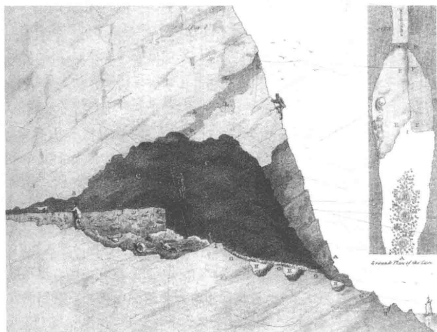
图2 帕夫兰的山羊洞穴(Goat's Hole cave, Paviland) 位于高尔南部海岸。红色女士(Red Lady)是在这里被发现的。这幅插图出现在威廉·巴克兰德(1784—1865年)1823年所著的《洪水的证据》一书中。在书中,他认为地球表面曾经被大洪水所淹没。这幅画是帕夫兰洞穴的平面和截面图。(威尔士国立图书馆)
