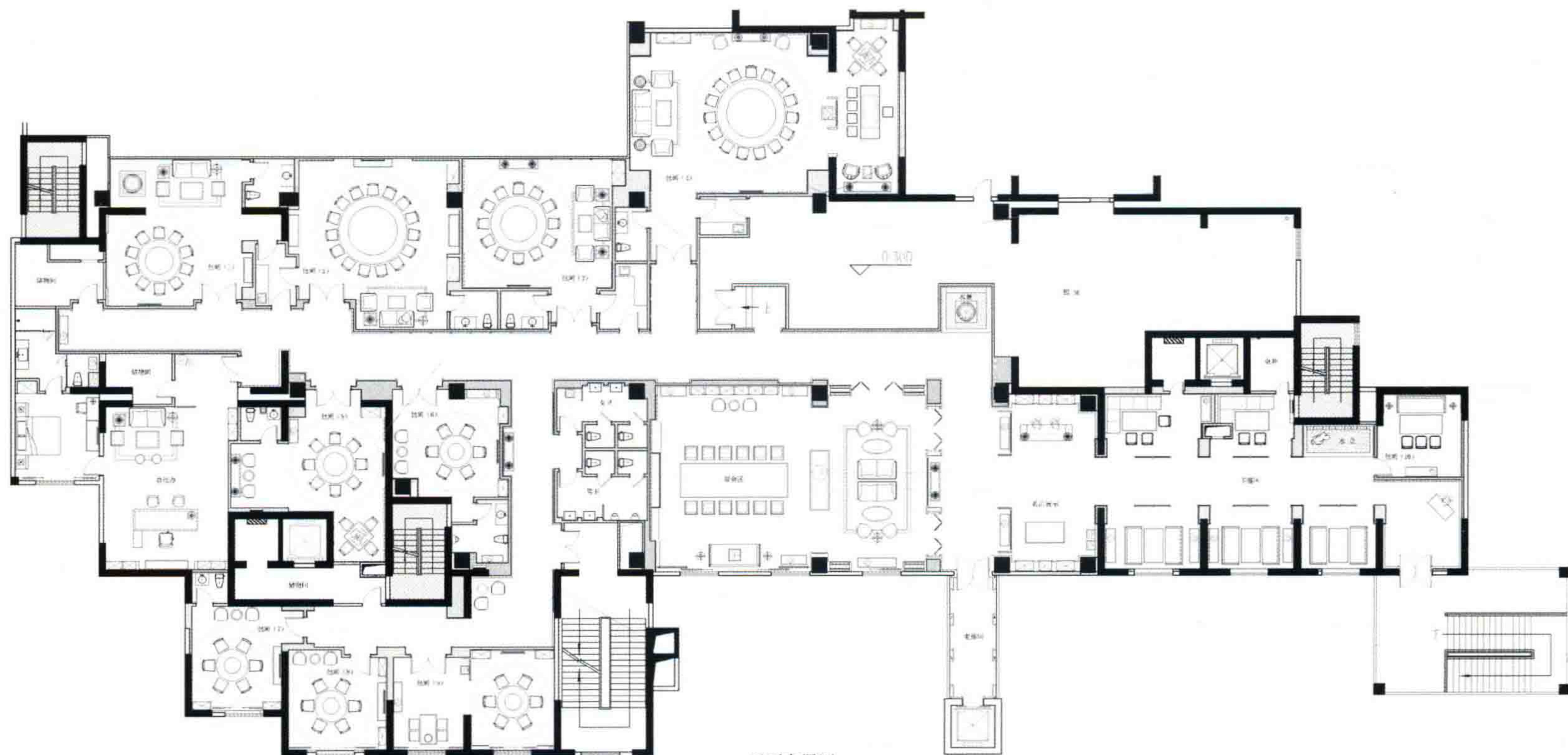
平面布置图
