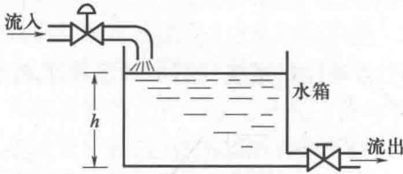
图 1-1 水箱液面
