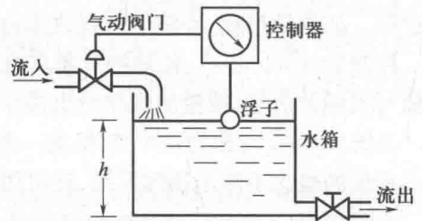
图 1-3 液面自动控制
