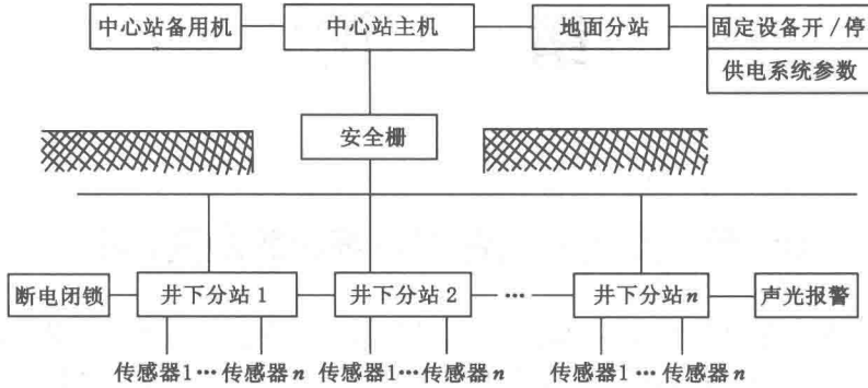
图 1-1 监测监控系统的组成
