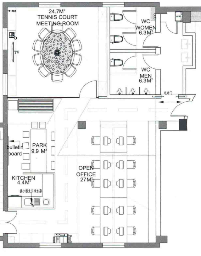
一层平面图
