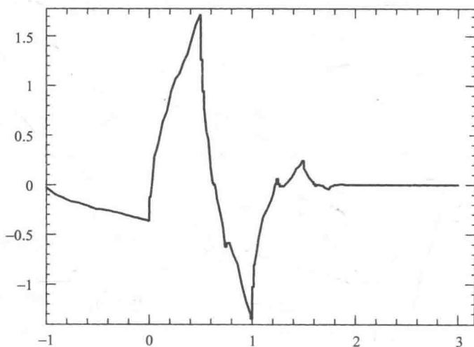
图4 Daubechies 小波
