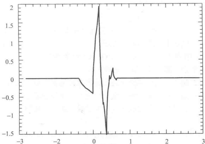
图 5 高频 Daubechies 小波
