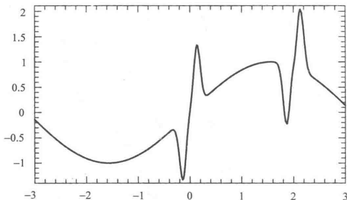
图3 具有孤立噪声的信号
