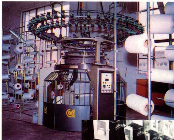
宏丽集团 GC-32F 纬编提花 大圆机
