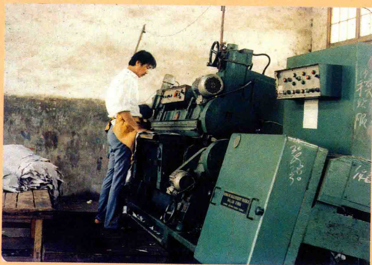
原高安皮革厂制革车间 (片皮工序)
